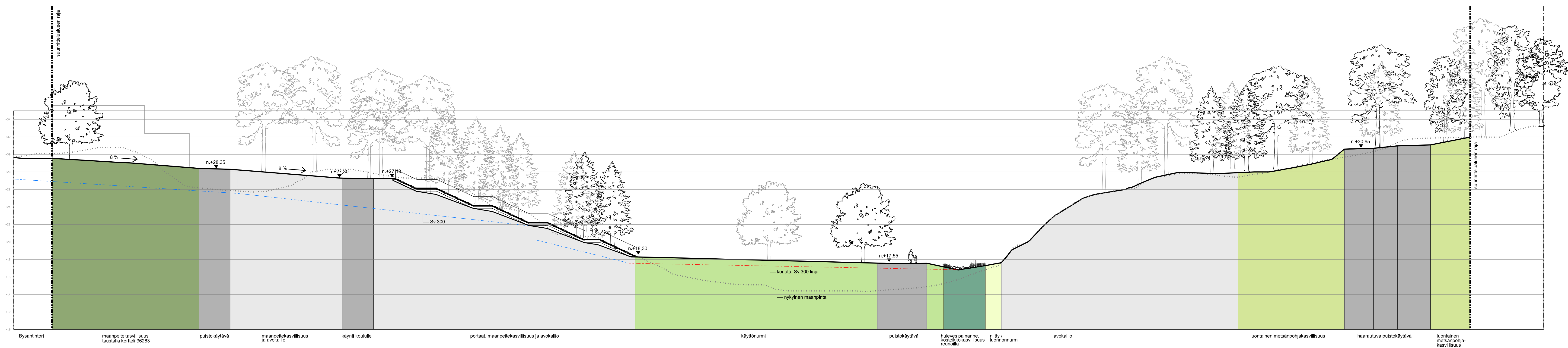
LEIKKAUS C - C'
