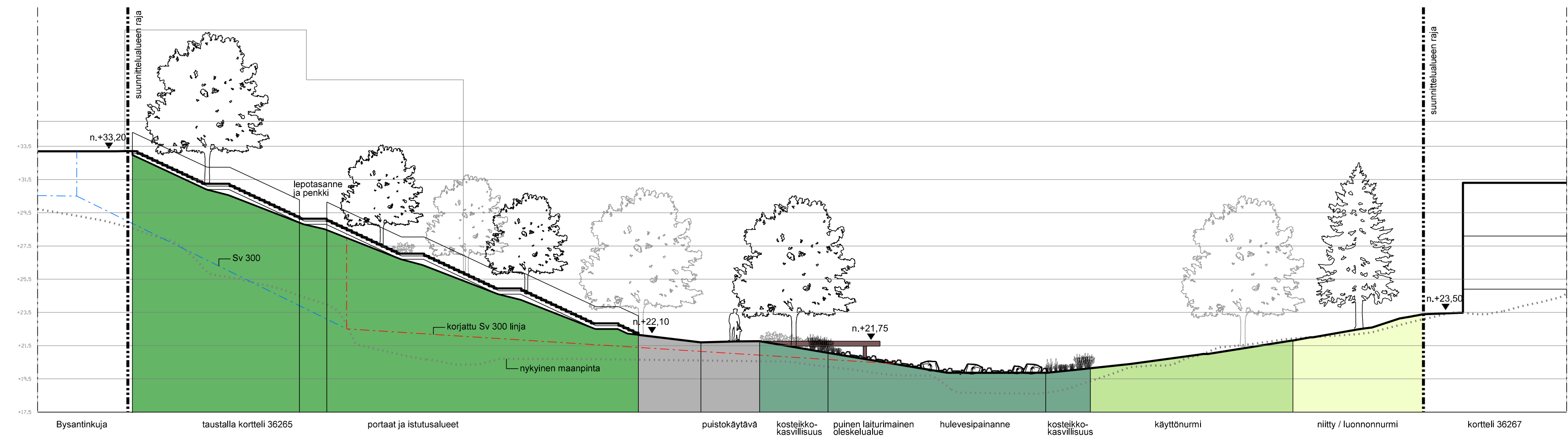
LEIKKAUS B - B'
