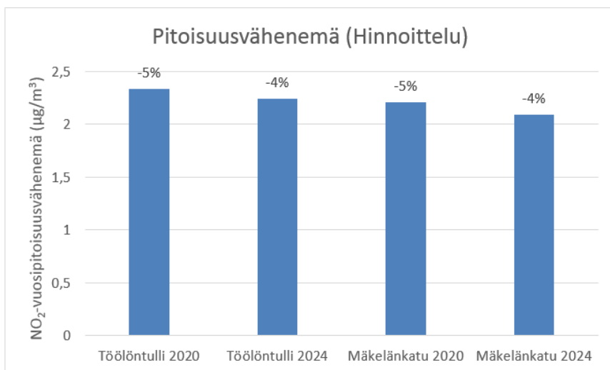
Kuva 14. Ajoneuvoliikenteen hinnoitteluskenaarion (toimenpide L1.2) arvoitu NO 2 -pitoisuusvähenemä nykytilaan (v. 2015) verrattuna vuosina 2020 ja 2024 kantakaupungin katukuilussa (Aarnio ym. 2016).
