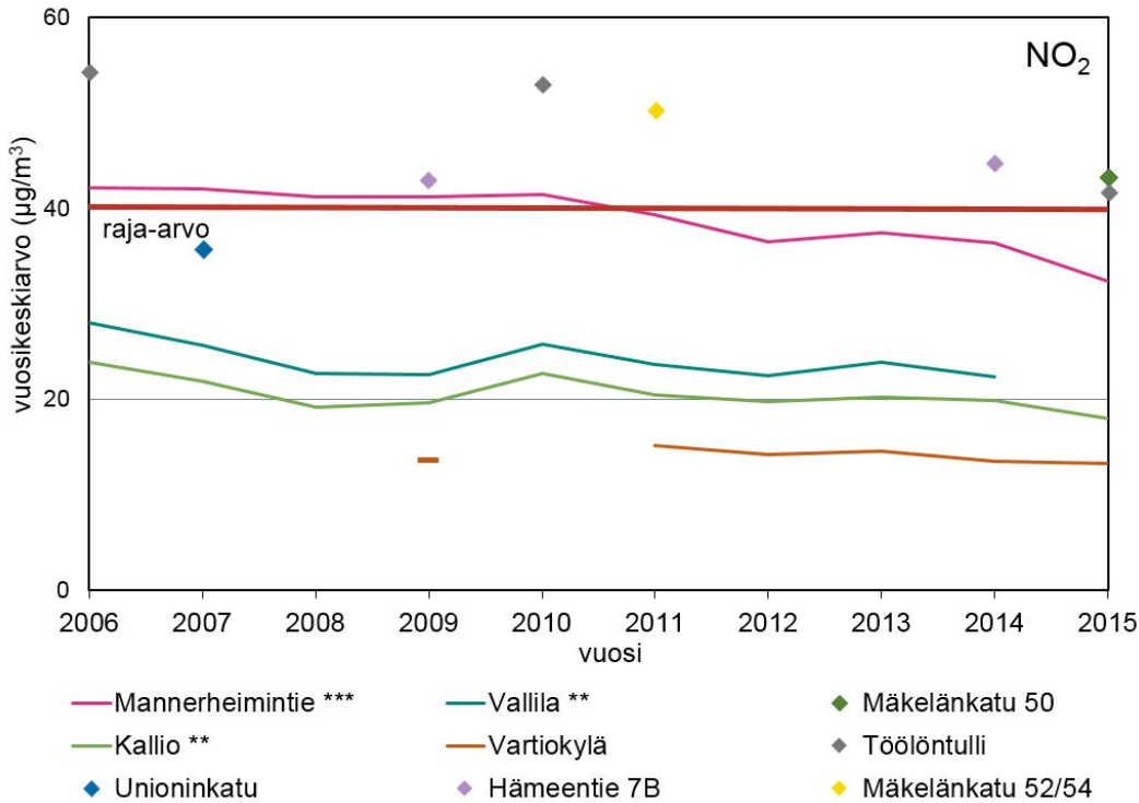
Kuva 1. Typpidioksidipitoisuuden vuosikeskiarvot ( \mu\text{g}/\text{m}^3 ) Helsingin jatkuvatoimisilla mittausasemilla (vasemmalla) Pitoisuusmuutosten tilastollinen merkitsevyystaso on laskettu vuosille 2001–2015: * pitoisuuden lasku melkein merkitsevä, ** merkitsevä, *** erittäin merkitsevä.
