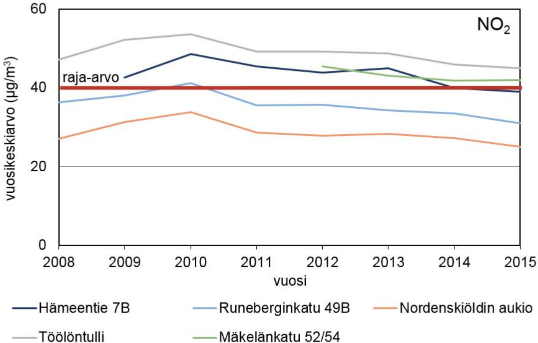
Kuva 2. Typpidioksidipitoisuuden vuosikeskiarvot ( \mu\text{g}/\text{m}^3 ) passiivikeräinkartoituksissa vuosina 2008–2015. Passiivikeräinkartoituksissa mittausarjat ovat liian lyhyitä trendien tilastollisen merkitsevyyden arvioimiseen.
