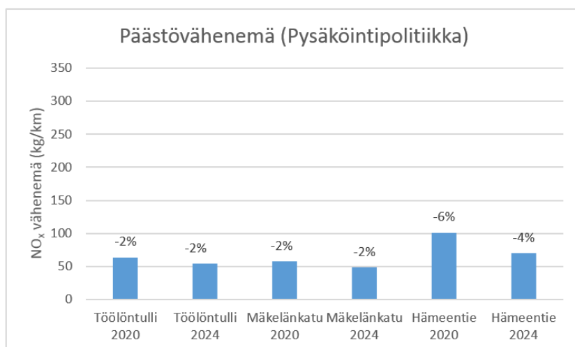
Kuva 19. Pysäköintipolitiikkaskenaarion (toimenpide L4.1) arvoitu NO x -päästövähennelmä nykytilaan (v. 2015) verrattuna vuosina 2020 ja 2024 kantakaupungin katukuilussa (Aarnio ym. 2016)
