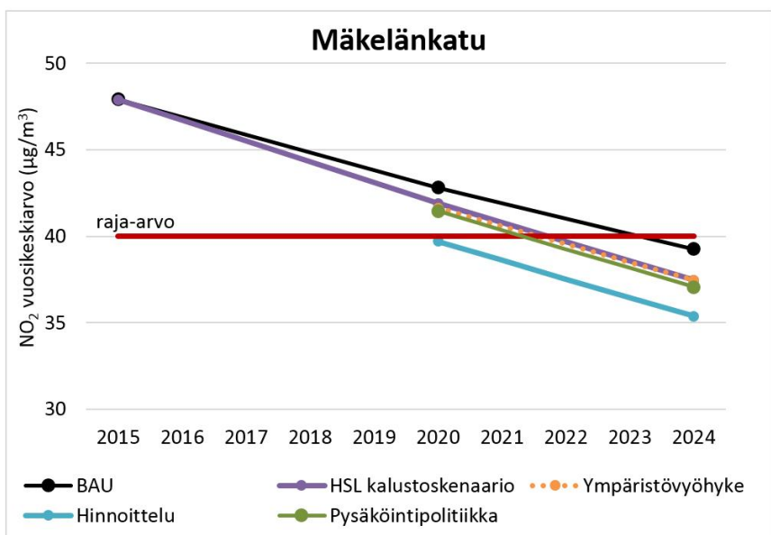
Kuva 5. Typpidioksidipitoisuuksien kehitys eri skenaarioissa (Aarnio ym. 2016) mallinnuksen mukaan vuoteen 2024 Mäkelänkadulla (Mäkelänkatu 50).
