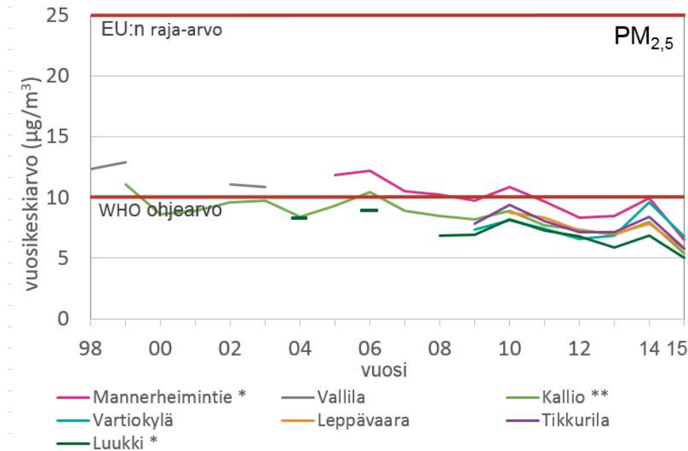
Kuva 9. Pienhiukkasten pitoisuudet ovat WHO:n ohjearvon tuntumassa sekä liikenneympäristöissä että pientaloalueilla. Pitoisuusmuutosten tilastollinen merkitsevyystaso on luokiteltu vuosille 2001–2015 kolmeen tasoon: * melkein merkitsevä, ** merkitsevä, *** erittäin merkitsevä. Kallion kaupunkitausta- asemalla pitoisuuden lasku on tilastollisesti merkitsevä. Mannerheimintien mittausasemalla ja Luukin alueellisella tausta- asemalla pitoisuuden lasku on tilastollisesti melkein merkitsevä. (Lähde: HSY)
