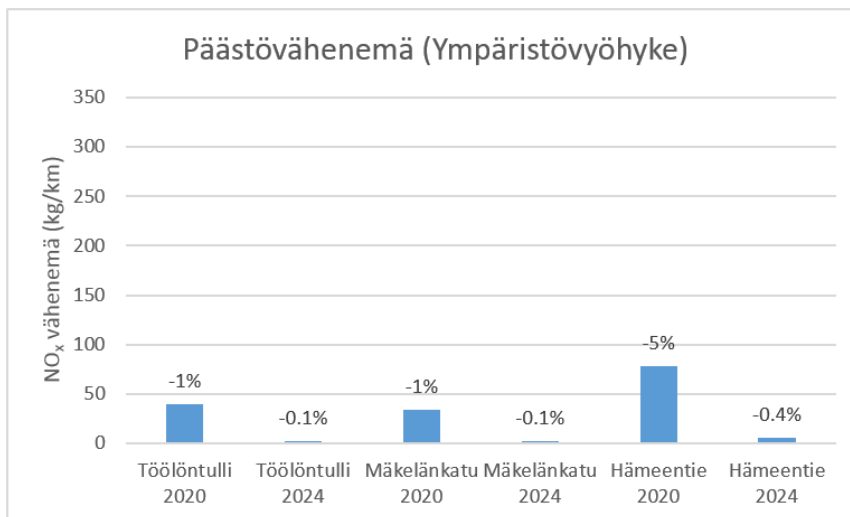
Kuva 17. Ympäristövyöhykeskenaarion (toimenpide L3.1) arvoitu \text{NO}_x -päästövähennys nykytilaan (v. 2015) verrattuna vuosina 2020 ja 2024 kantakaupungin katukuiluissa (Aarnio ym. 2016).
