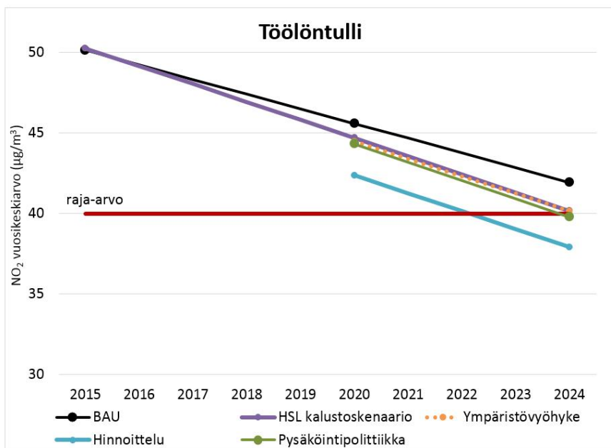
Kuva 4. Typpidioksidipitoisuuksien kehitys eri skenaarioissa mallinnuksen mukaan (Aarnio ym. 2016) vuoteen 2024 Töölöntullissa (Mannerheimintie 55).
