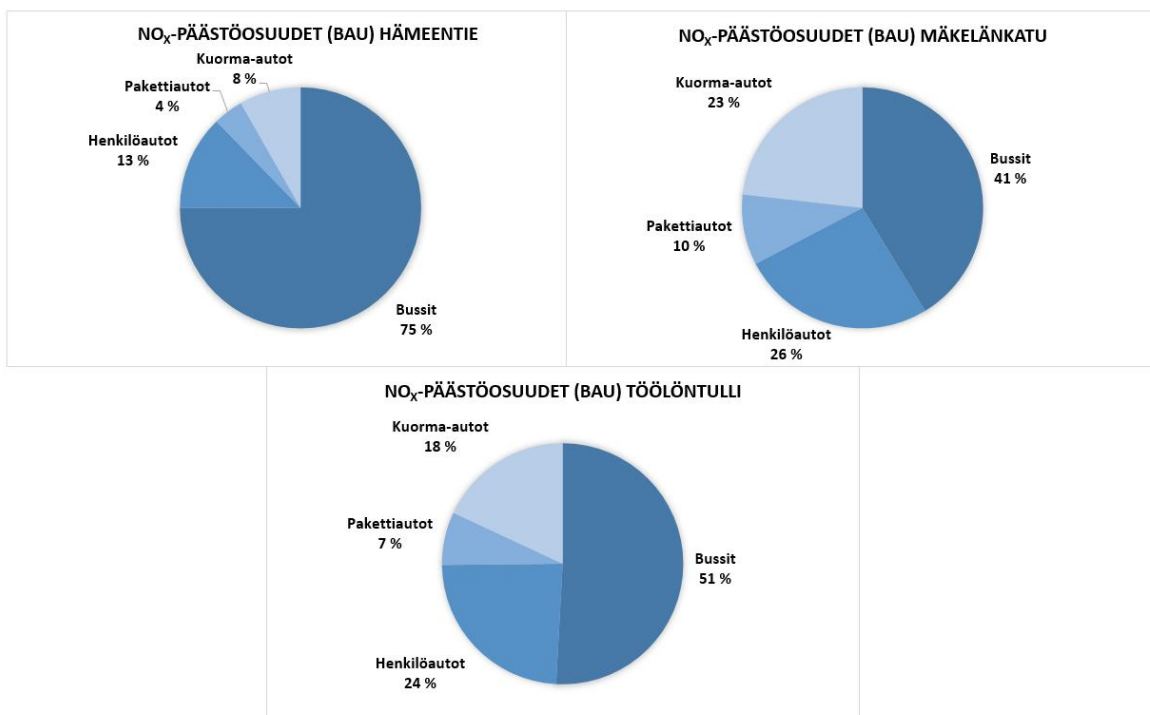
Kuva 12. Henkilöautojen, pakettiautojen, bussien ja kuorma-autojen päästöosuudet ilman toimenpiteitä (BAU) Mäkelänkadulla, Hämeentiellä ja Töölöntullissa vuonna 2015 (Aarnio ym. 2016).
