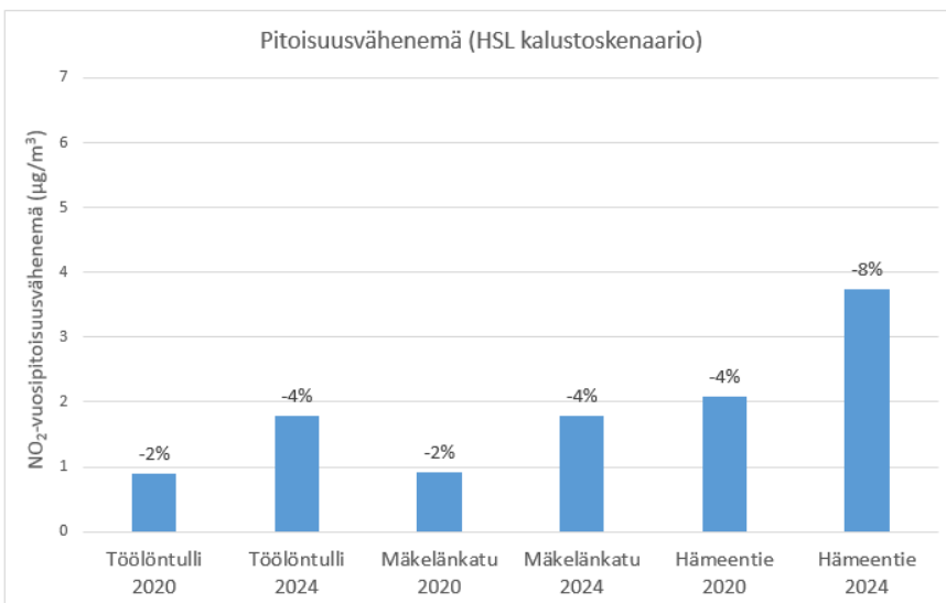
Kuva 16. HSL:n kalustoskenaarion (toimenpide L2.1) arvoitu NO 2 -pitoisuusvähenemä nykytilaan (v. 2015) verrattuna vuosina 2020 ja 2024 kantakaupungin katukäytävillä (Aarnio ym. 2016).
