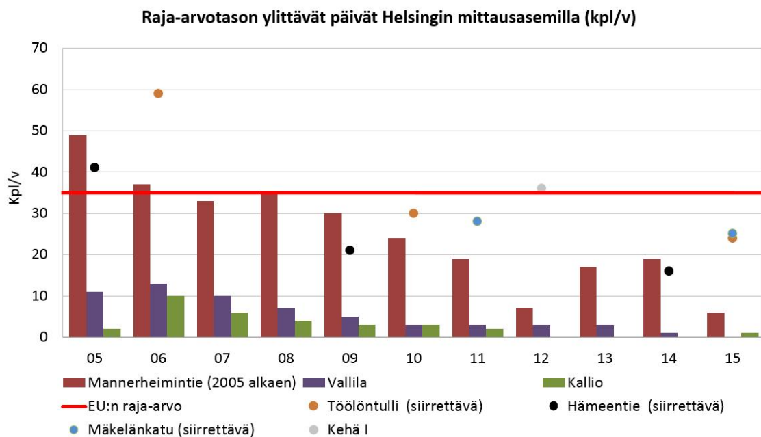
Kuva 21. Vuorokausiraja-arvotason (50 µg/m 3 ) ylittävät päivät Helsingin mittausasemilla (kpl/v) vuosina 2005–2015. (Kuvan tiedot HSY)
