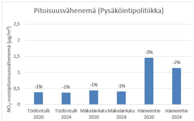
Kuva 20. Pysäköintipolitiikkaskenaarion (toimenpide L4.1) arvoitu NO 2 -pitoisuusvähenemä nykytilaan (v. 2015) verrattuna vuosina 2020 ja 2024 kantakaupungin katukuilussa (Aarnio ym. 2016).
