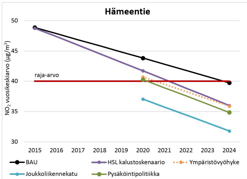
Kuva 6. Typpidioksidipitoisuuksien kehitys eri skenaarioissa (Aarnio ym. 2016) mallinnuksen mukaan vuoteen 2024 Hämeentiellä (Hämeentie 7).
