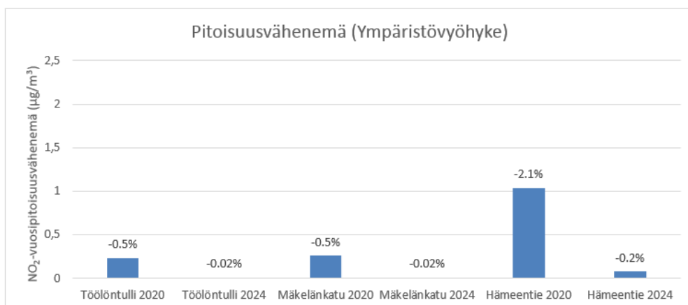
Kuva 18. Ympäristövyöhykeskenaarion (toimenpide L3.1) arvoitu NO 2 -pitoisuusvähennelmä nykytilaan (v. 2015) verrattuna vuosina 2020 ja 2024 kantakaupungin katukuilussa (Aarnio ym. 2016).
