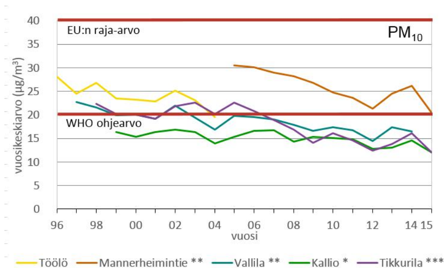
Kuva 22. Hengitettävien hiukkasten vuosipitoisuudet pääkaupunkiseudun mittausasemilla vuosina 1996 – 2015. Pitoisuusmuutosten tilastollinen merkitsevyytaso on luokiteltu vuosille 2001–2014 kolmeen tasoon: * melkein merkitsevä, ** merkitsevä, *** erittäin merkitsevä. Tikkurilan mittausasemalla pitoisuuden lasku on tilastollisesti erittäin merkitsevä. Mannerheimintien ja Vallilan mittausasemilla pitoisuuden lasku on tilastollisesti merkitsevä ja Kallion kaupunkitausta- asemalla tilastollisesti melkein merkitsevä. (Kuva HSY)
