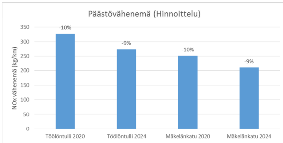
Kuva 13. Ajoneuvoliikenteen hinnoitteluskenaarion (toimenpide L1.2) arvioitu NO x -päästövähennelmä nykytilaan (v. 2015) verrattuna vuosina 2020 ja 2024 kantakaupungin katukuilussa (Aarnio ym. 2016).
