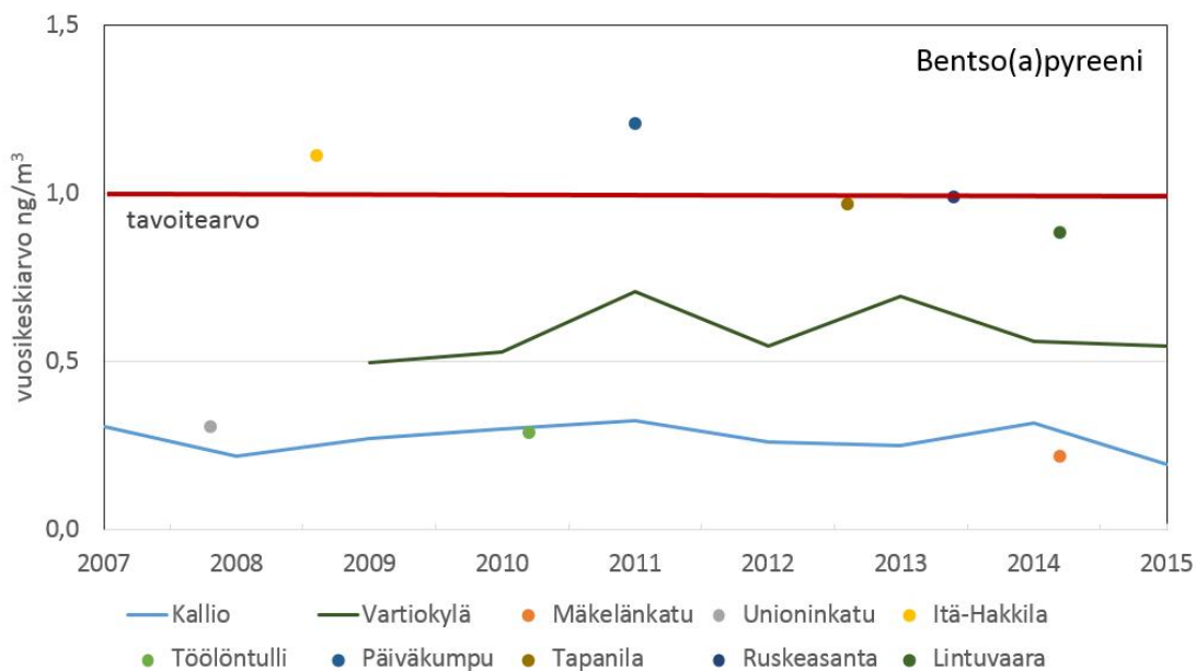
Kuva 26. Bentso(a)pyreenin vuosipitoisuudet ylittävät paikoitellen tavoitearvon pääkaupunkiseudulla (Malkki ja Loukkola 2014).
