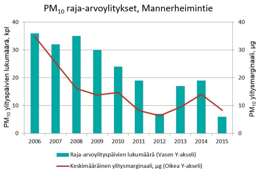
Kuva 23. Vuorokausiraja-arvotason ( 50 \mu\text{g}/\text{m}^3 ) ylittävät päivät Mannerheimintien mittausasemalla (kpl/v, palkit) ja ylityspäivien keskimääräinen ylitysmarginaali ( \mu\text{g}/\text{m}^3 , viiva). (Kuvan tiedot HSY)
