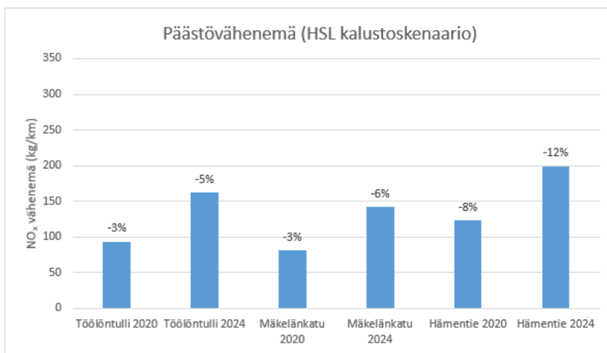
Kuva 15. HSL:n kalustoskenaarion (toimenpide L2.1) arvoitu NO x -päästövähennelmä nykytilaan (v. 2015) verrattuna vuosina 2020 ja 2024 kantakaupungin katukäytävillä (Aarnio ym. 2016).
