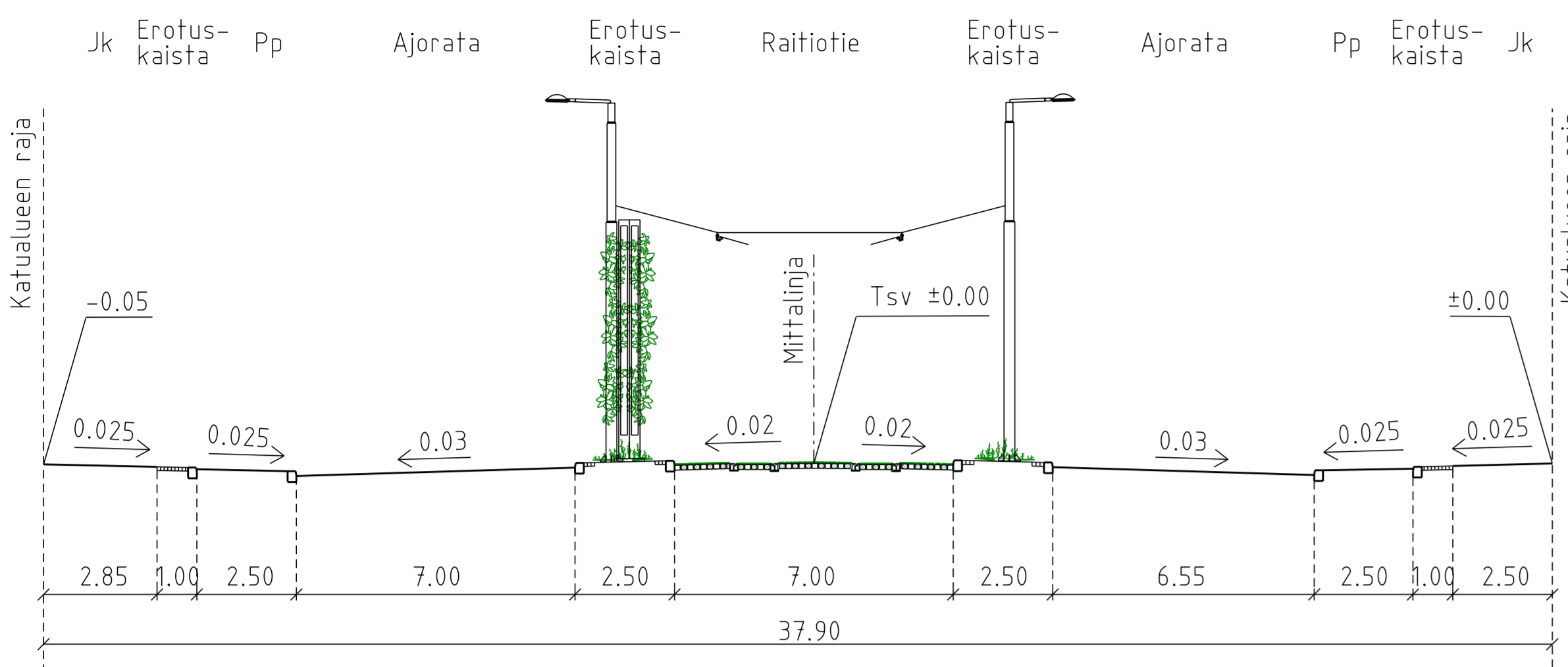
POIKKILEIKKAUS A-A 1:200
