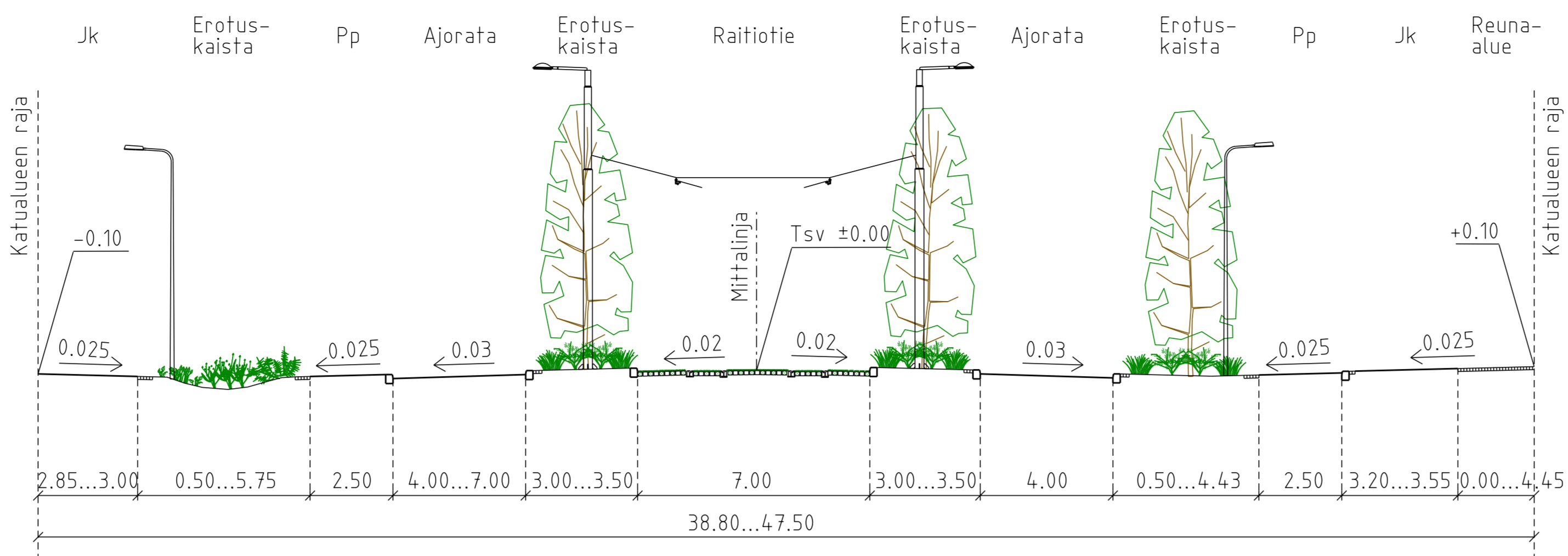
POIKKILEIKKAUS B-B 1:200
