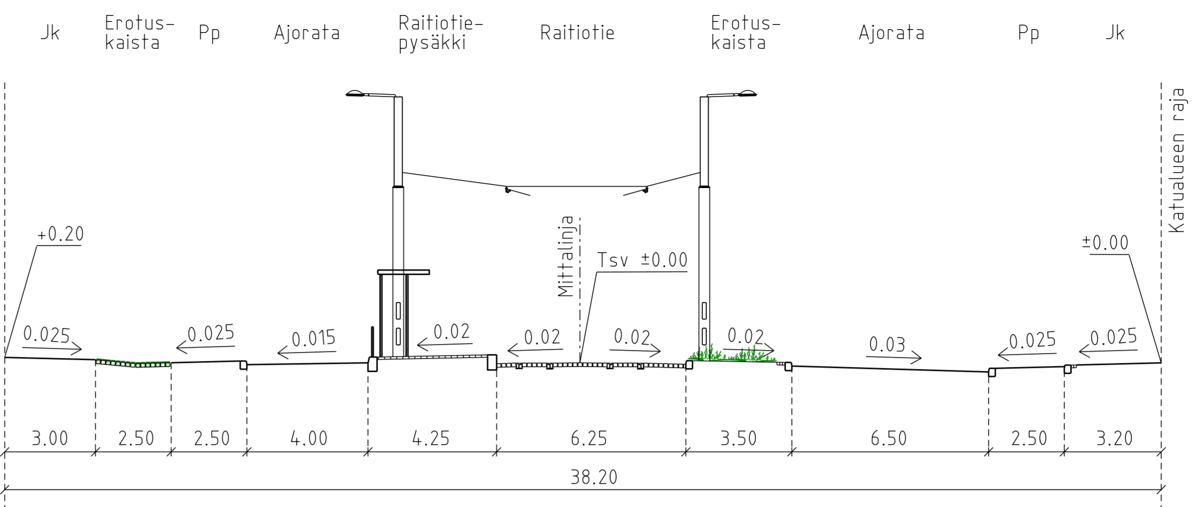
POIKKILEIKKAUS C-C 1:200
