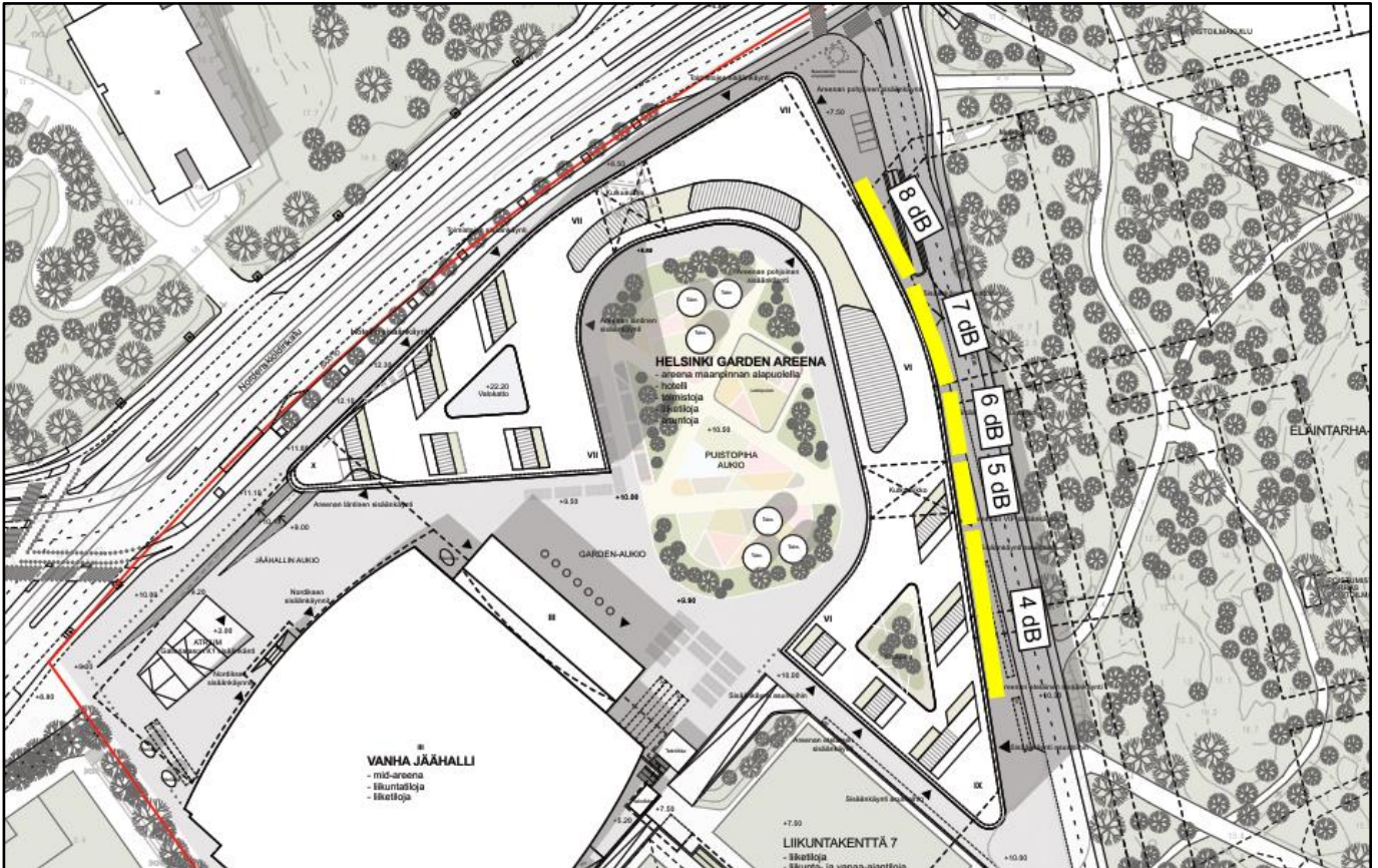
Kuva 11. Suositukset parvekejulkisivujen ääneneristysvaatimuksiksi. \Delta L_{A,vaad} 3 dB ja sitä pienemmät vaatimukset täyttyvät tavanomaisella lasituksella.
