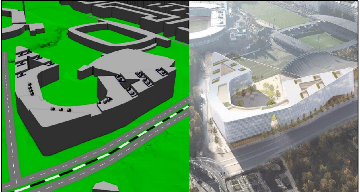
Kuva 3. Mallinnettu tilanne (vas.) sekä arkkitehdin havaintokuva kattoterasseista (oik)
