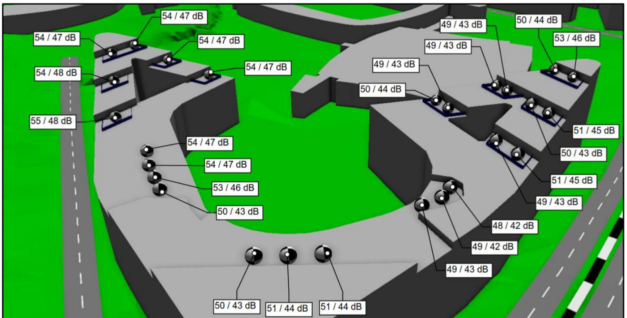
Kuva 4. Vuoden 2040 ennustetilanteen keskiäänitasot L_{A,eq} kattoterassilla (päiväaika / yöaika)
