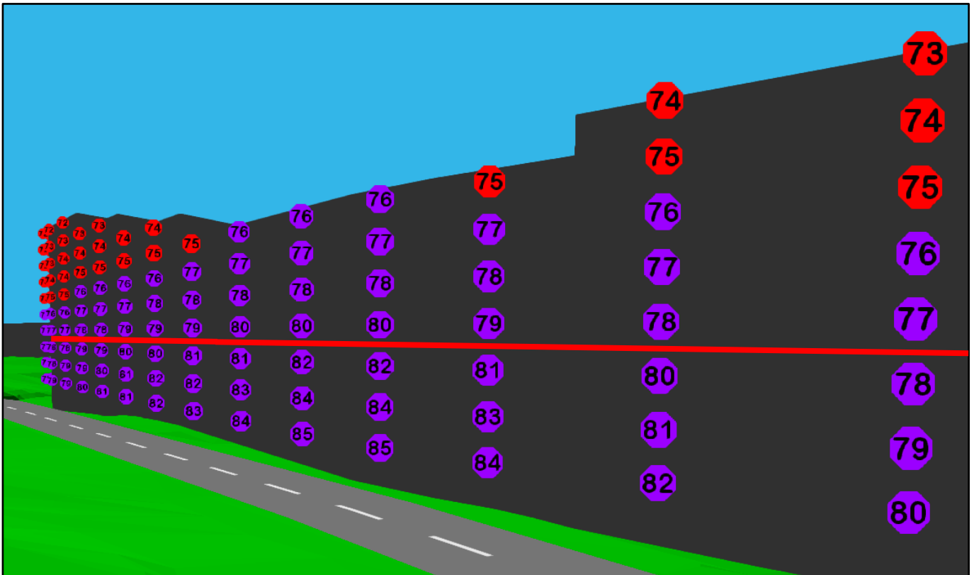
Kuva 7. Raskaan liikenteen enimmäisäänitasot L_{A,F,max} itäjulkisivulla. Suurimmat äänitasot sijaitsevat aivan itäisen kulkuaukon pohjoispuolella. Alin asuinkerros (3. krs) sijaitsee viitesuunnitelman mukaan punaisen viivan yläpuolella (lattiakorko +19,20)
