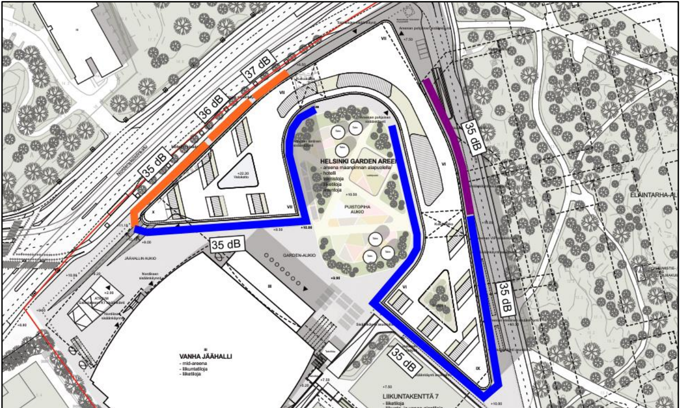
Kuva 16. Suositukset ulkovaipan ääneneristysvaatimuksiksi \Delta L_{A,vaad} . Oranssilla värjätyt vaatimukset muodostuvat liikenteen keskiäänitasoista, violetilla värjätyt liikenteen enimmäisäänitasoista ja sinisellä värjätyt kohdassa 6 esitetyistä muista melulähteistä.
