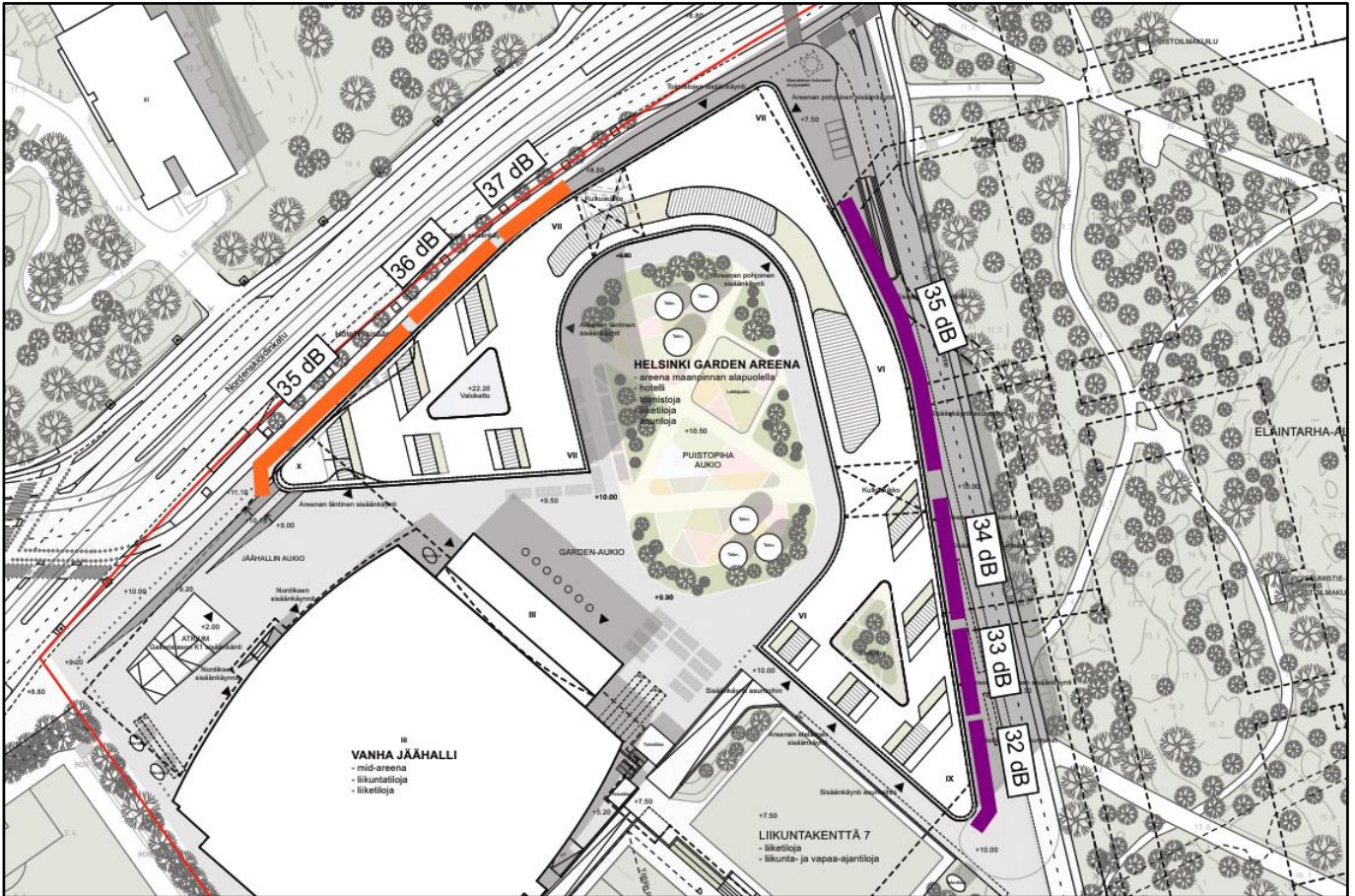
Kuva 10. Suositukset ulkovaipan ääneneristysvaatimuksiksi \Delta L_{A,vaad} . Keskiäänitasoista muodostuvat vaatimukset on värjätty oranssilla ja enimmäisäänitasoista muodostuvat vaatimukset violetilla.
