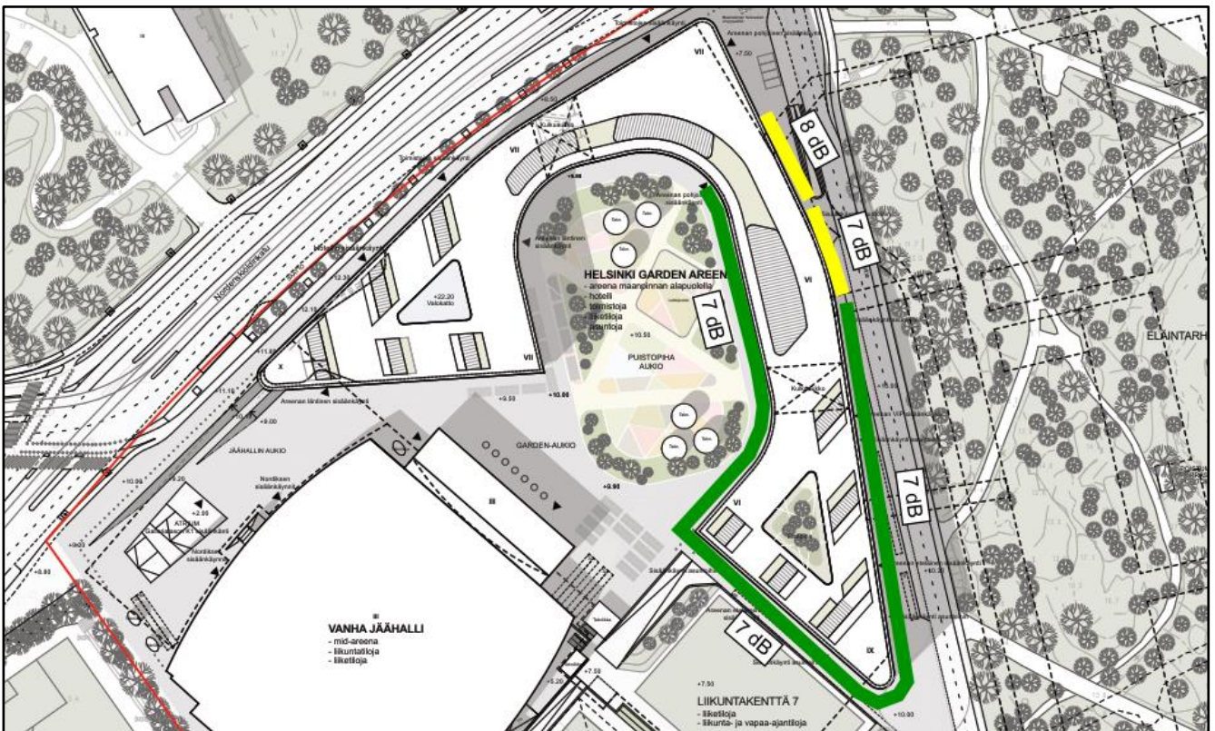
Kuva 17. Suositukset parvekeulkisivujen ääneneristysvaatimuksiksi \Delta L_{A,vaad} . Keltaisella värjätyt vaatimukset muodostuvat liikenteen keskiäänitasoista ja vihreällä värjätyt vaatimukset kohdassa 6 esitetyistä muista melulähteistä.
