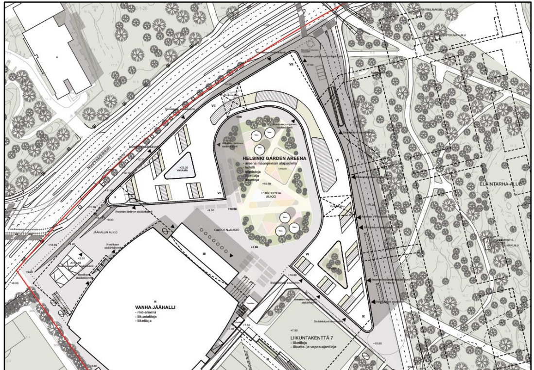
Kuva 1. Kohteen Garden Helsinki viitesuunnitelman asemapiirustus
