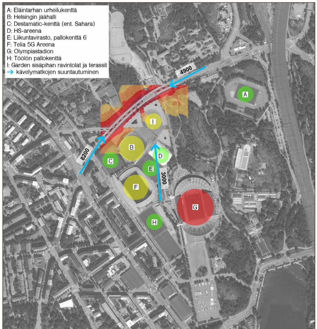
Kuva 12: Kohteen ympäristössä alle 500 m etäisyydellä sijaitsevat mahdolliset melulähteet. Melulähteet on väritetty niiden vaikuttavuuden mukaan (punainen = merkittävä melulähde, keltainen = toissijainen melulähde, vihreä = vähäinen melulähde). Kuva: Google Maps.
