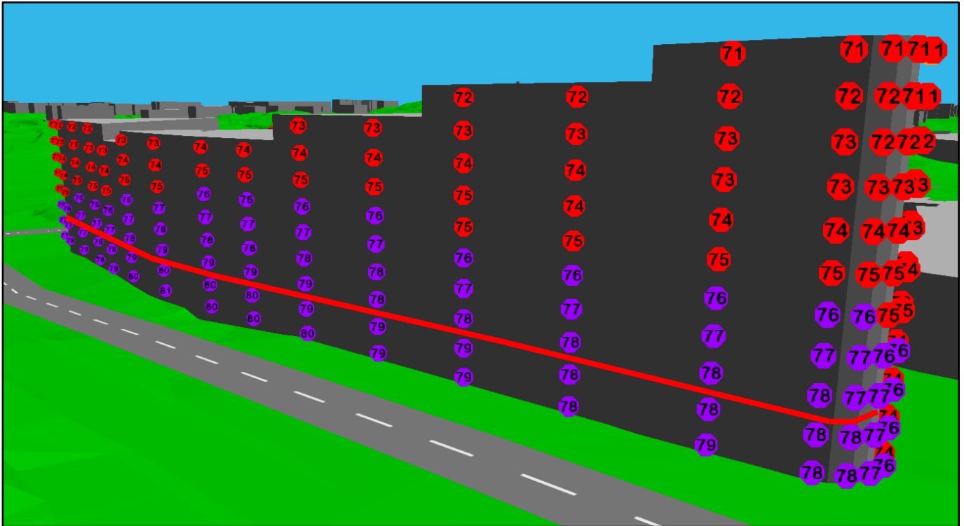
Kuva 8. Raskaan liikenteen enimmäisäänitasot L_{A,F,max} pohjoisjulkisivulla. Julkisivulla ei sijaitse asuntoja. Alimmat hotellihuoneet sijaitsevat viitesuunnitelman mukaan punaisen viivan yläpuolella (lattiakorko +12,70)
