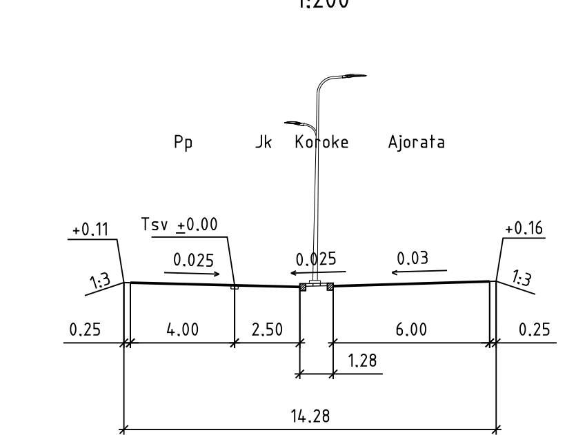
POIKKILEIKKAUS C-C 1:200
