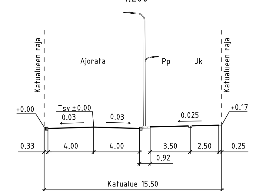
POIKKILEIKKAUS B-B 1:200
