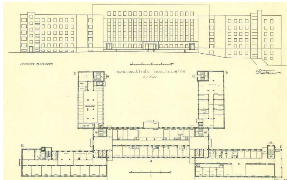
PÄÄRAKENNUKSEN POHJOISJULKISIVU 1-KERROKSEN POHJAPIIRUSTUS Arkkitehti Eino Forsman, 1941
