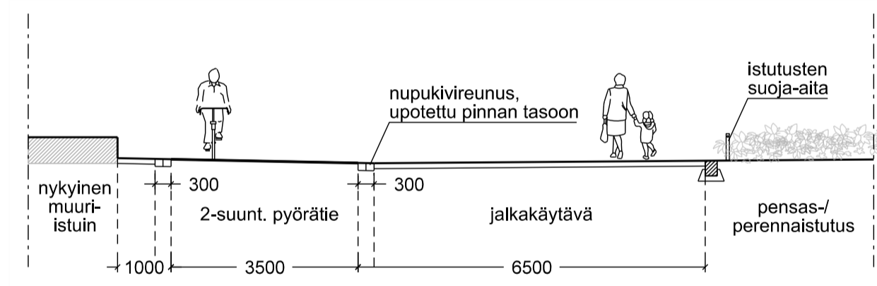
POIKKILEIKKAUS A - A' 1:100 JALANKULKU- JA PYÖRÄILYPROMENADI
