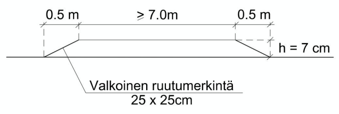
KOROTETTU SUOJATIE / KOROTETTU LIITTYMÄ POIKKILEIKKAUKSET 1:200
