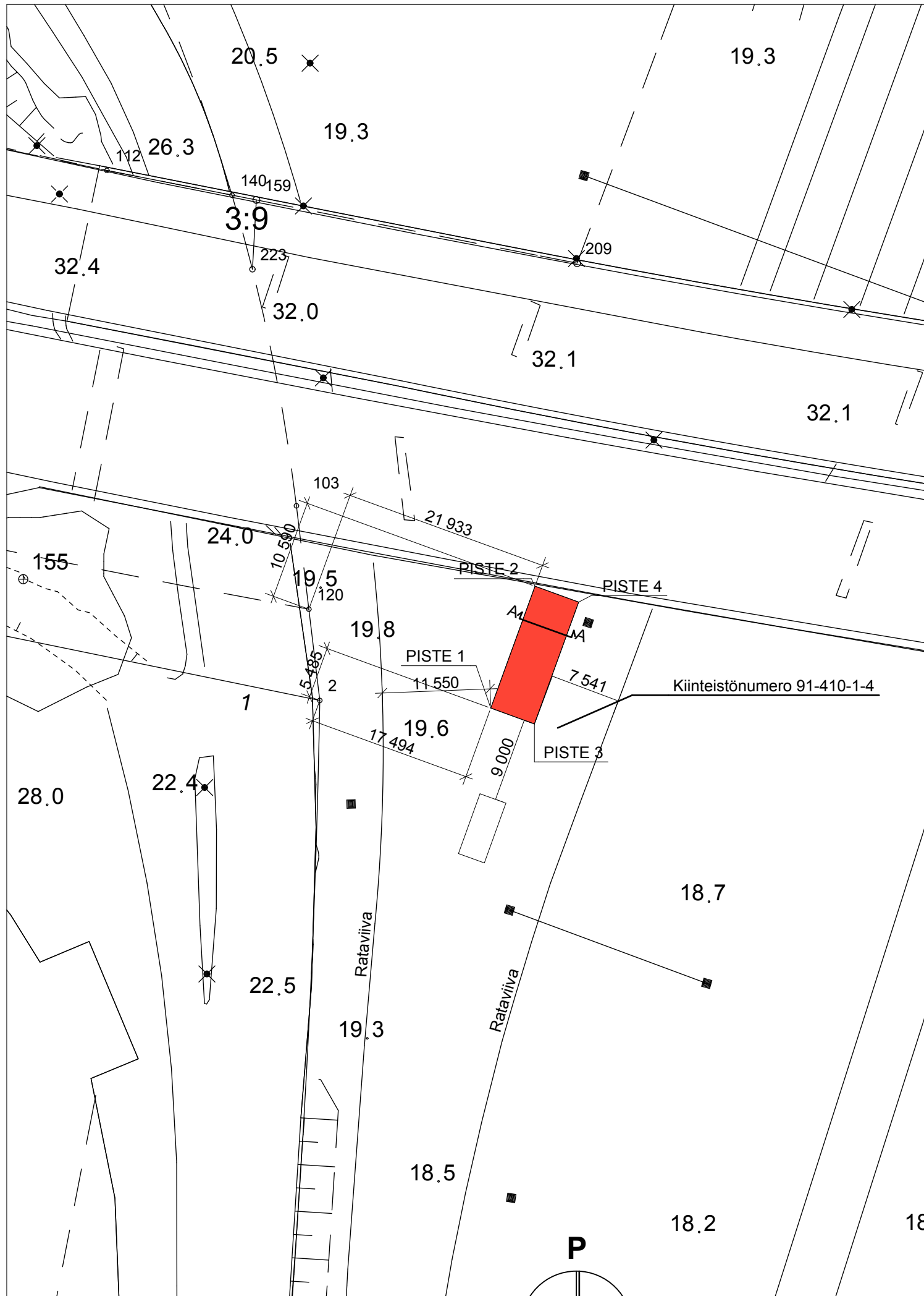
Asemapiirustus 1:500
