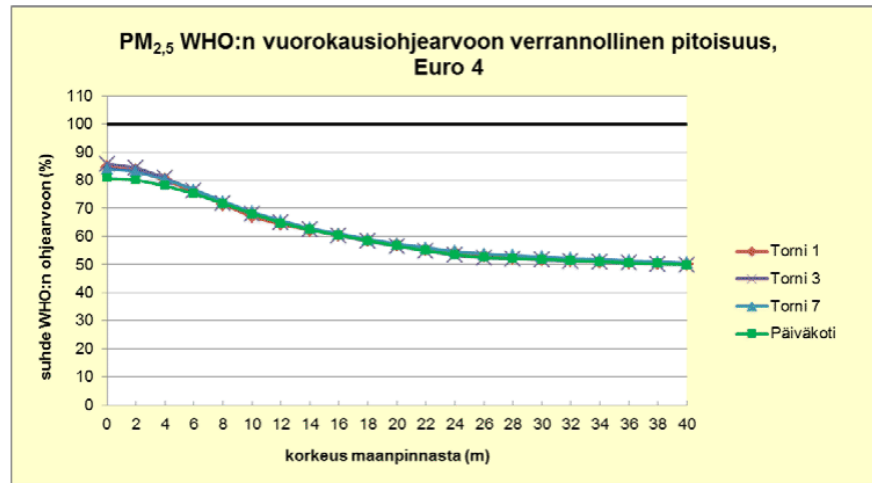
Kuva 16. Pienhiukkasten ( PM_{2.5} ) vuorokausiohjeeseen verrannollinen pitoisuus erillisissä eri korkeustasoilla Euro 4 -päästötasolla ja nykytilanteen liikennemäärillä laskettuna.
