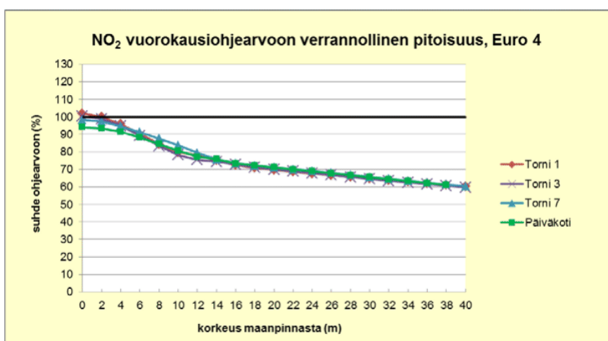
Kuva 12. Typpidioksidin (NO 2 ) vuorokausiohjeeseen verrannollinen pitoisuus erillispisteissä eri korkeustasoilla Euro 4 -päästötasolla ja nykytilanteen liikennemäärillä laskettuna.
