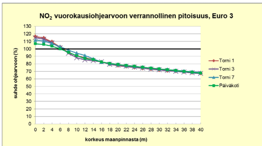
Kuva 11. Typpidioksidin (NO 2 ) vuorokausiohjeeseen verrannollinen pitoisuus erillispisteissä eri korkeustasoilla Euro 3 -päästötasolla ja nykytilanteen liikennemäärillä laskettuna.
