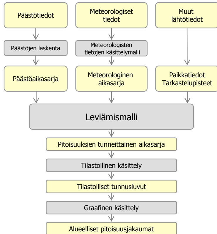
Kuva B. Kaaviokuva Ilmätieteen laitoksella kehitetyn leviämismallin, viivalähdemallin (CAR-FMI) toiminnasta.
