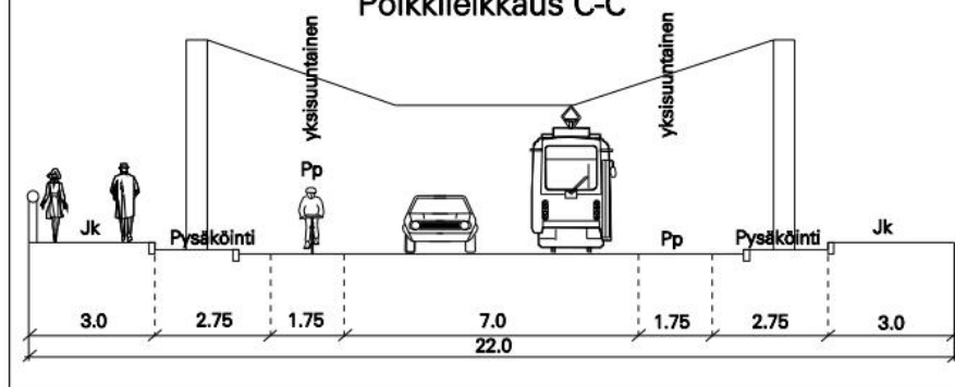
Poikkileikkaus C-C
