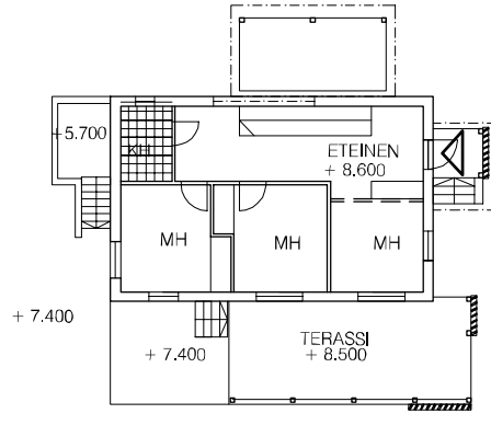
POHJAPIIRROS 1.KRS
