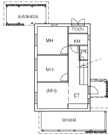
POHJAPIIRROS 1.KRS.
