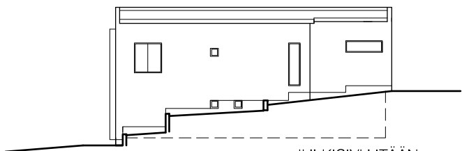
JULKISIVU ITÄÄN
