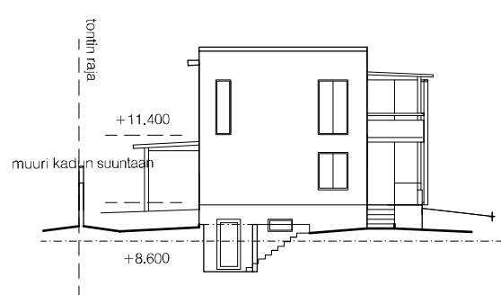
JULKISIVU LÄNTEEN
