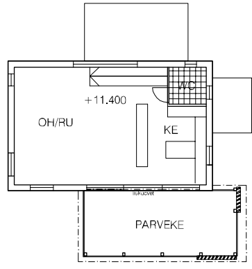
POHJAPIIRROS 2.KRS
