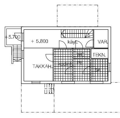
POHJAPIIRROS KELLARI
