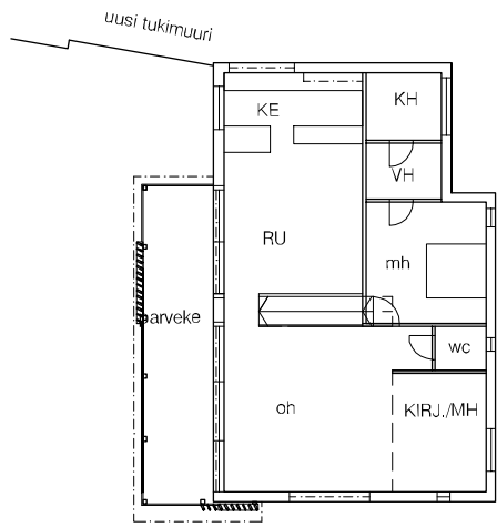
POHJAPIIRROS 2.KRS.
