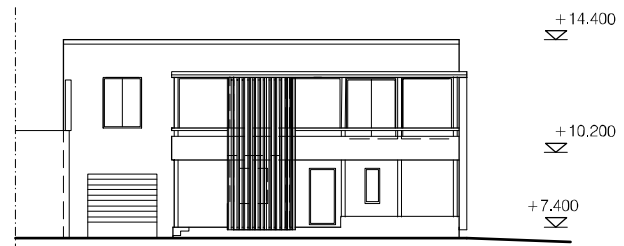
JULKISIVU LÄNTEEN
