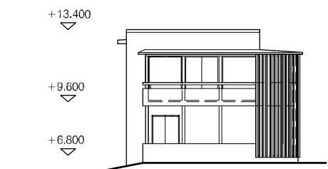
JULKISIVU ETELÄÄN
