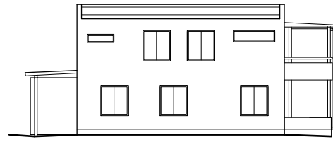
JULKISIVU LÄNTEEN
