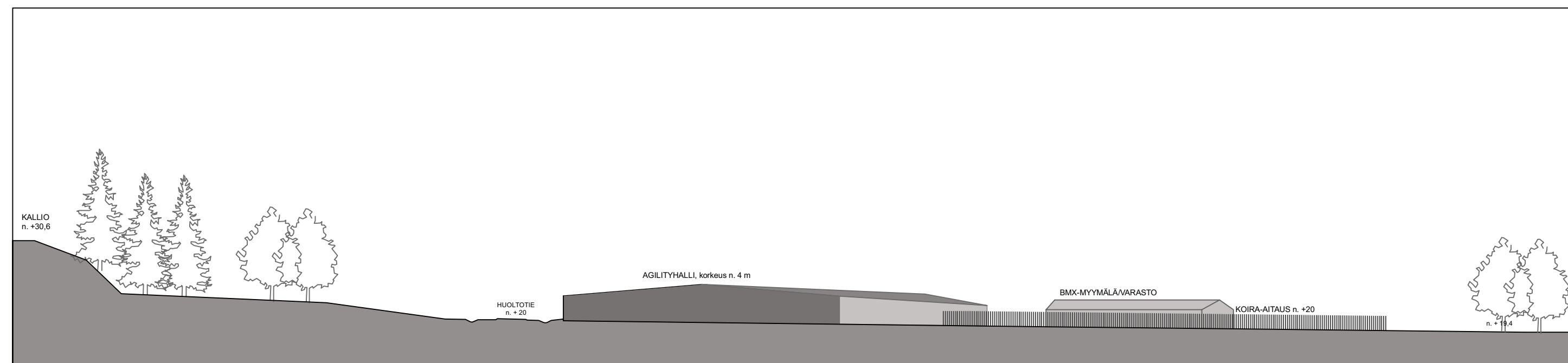
LEIKKAUS B-B' AGILITYHALLIN SUHTEESTA YMPÄRISTÖÖN 1:500
