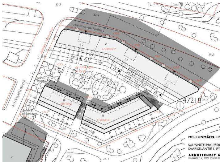
Pyhäntunturintie 2, viitesuunnitelma Arkkitehdit Mauri Korokka ja Kirsti Rantanen
