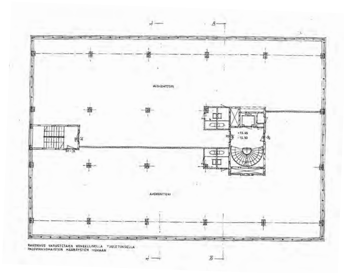
Rakennuksen 2. ja 3. kerroksen pohja
