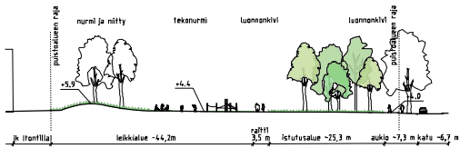
LEIKKAUS A-A 1:500
