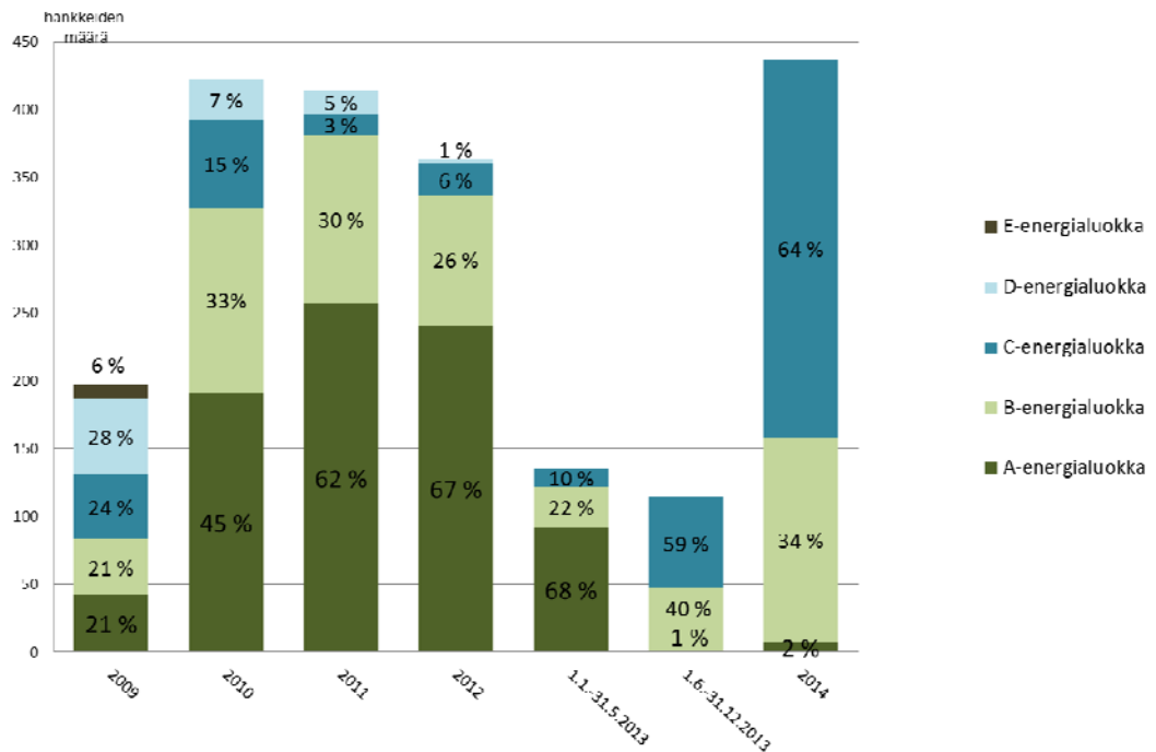
Kuva 15. Asuinrakennushankkeille myönnettyjen rakennuslupien energiatehokkuusluokat Helsingissä 2009–2014. Lähde: Rakennusvalvontavirasto.
