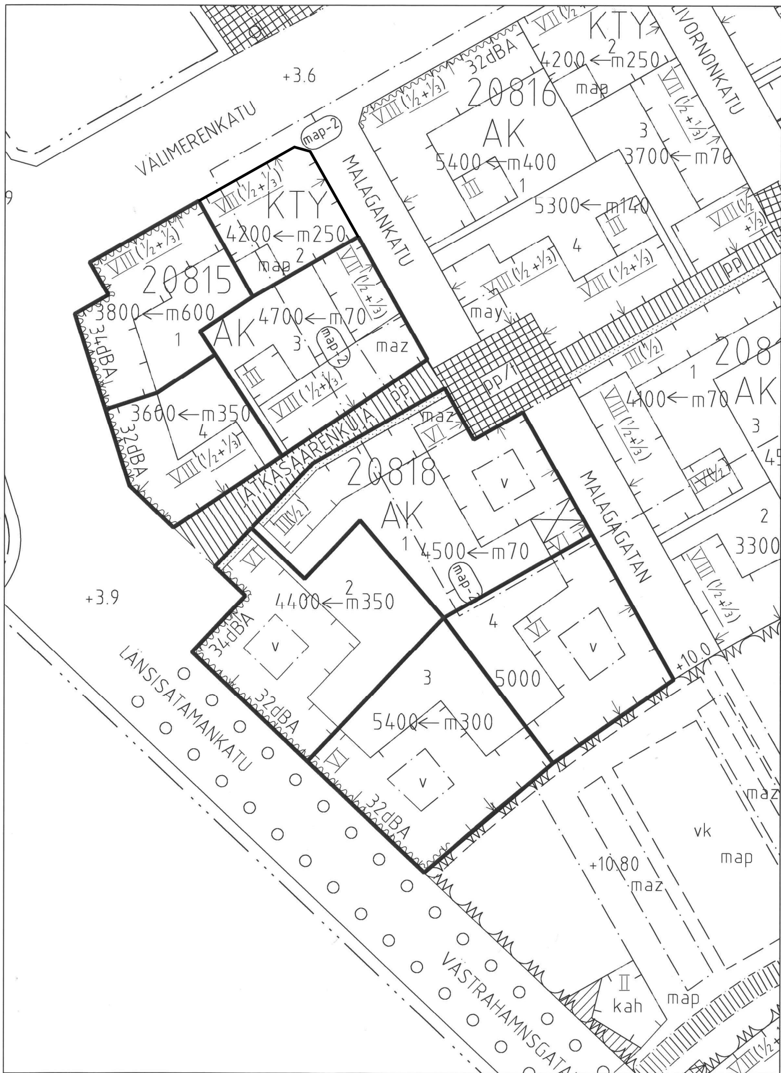
JÄTKÄSAARI Kortteli 20815 ja Kortteli 20818 Mittakaava 1:1000
