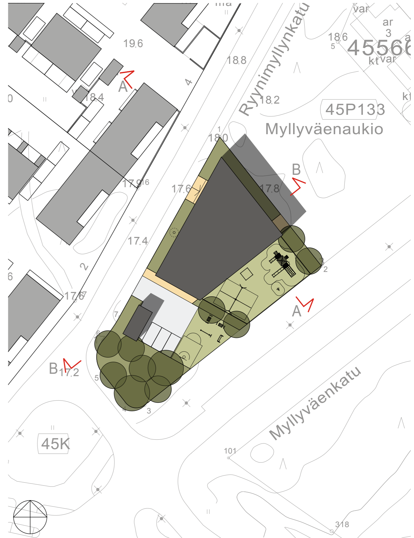
asemapiirros 1:500
