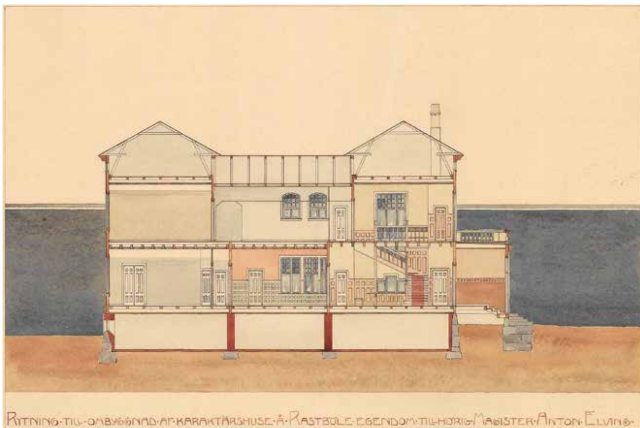
Kuva 13. Arkkitehti Birger Federleyn laatimassa päärakennuksen muutospiirustuksessa vuodelta 1908 terassit aukeavat etelään ja pihan keskeisenä aiheena on ruusuryhmä. Rakennuksen muutostyöt eivät toteutuneet. ARKMU.
