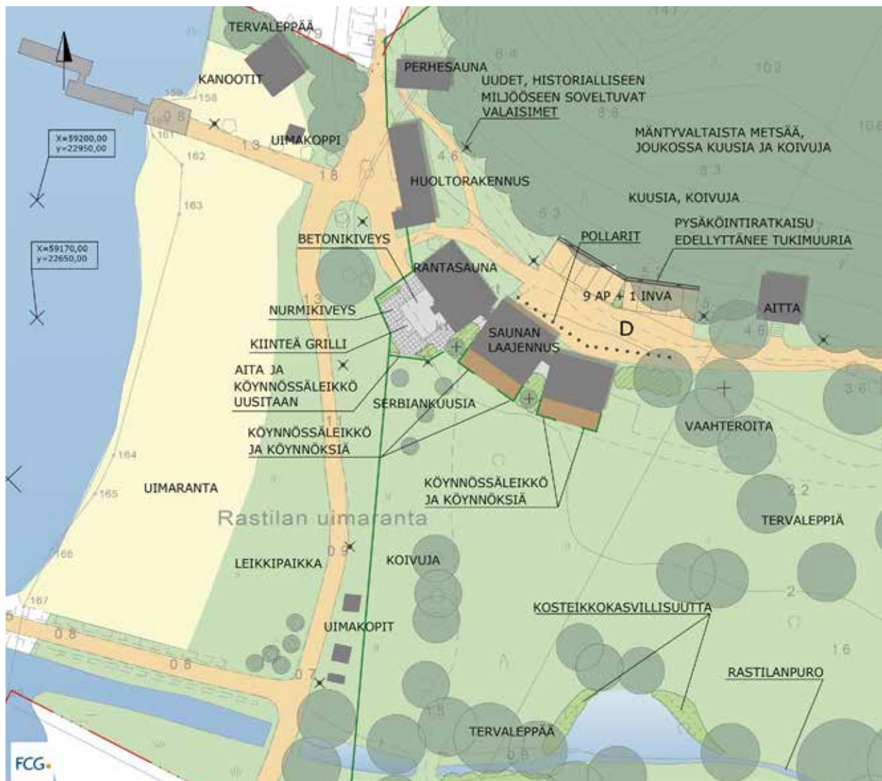
Kuva 36. Ote LT-Konsultit Oy:n laatimasta Rastilan leirintäalueen yleissuunnitelman tarkastuksesta vuodelta 2010 (HKT).
