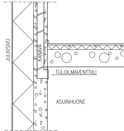
Tuloilmaventtiili kun julkisivuelementtejä on 1 / asuinhuone
