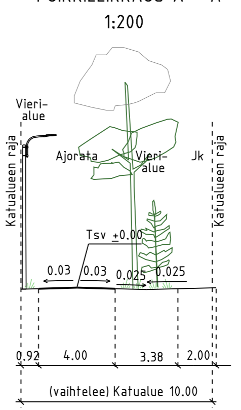
POIKKILEIKKAUS A - A 1:200
