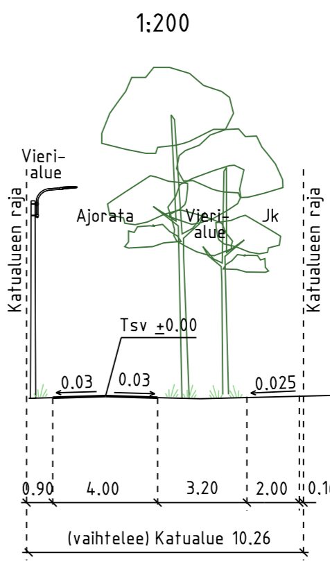
POIKKILEIKKAUS B - B 1:200
