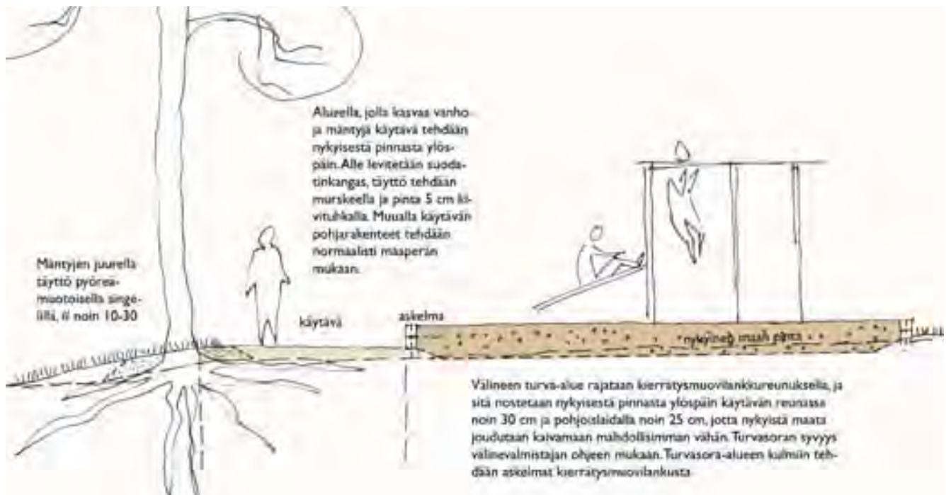
Periaateleikkaus käytävästä suurten mänttien alla ja kuntovälineen asentamisesta.
