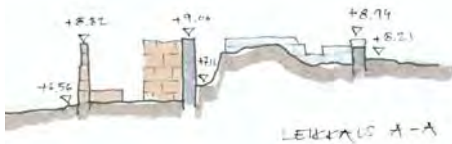
Gebhardin huvilan raunio nykyään, julkisivut ja leikkaus.
