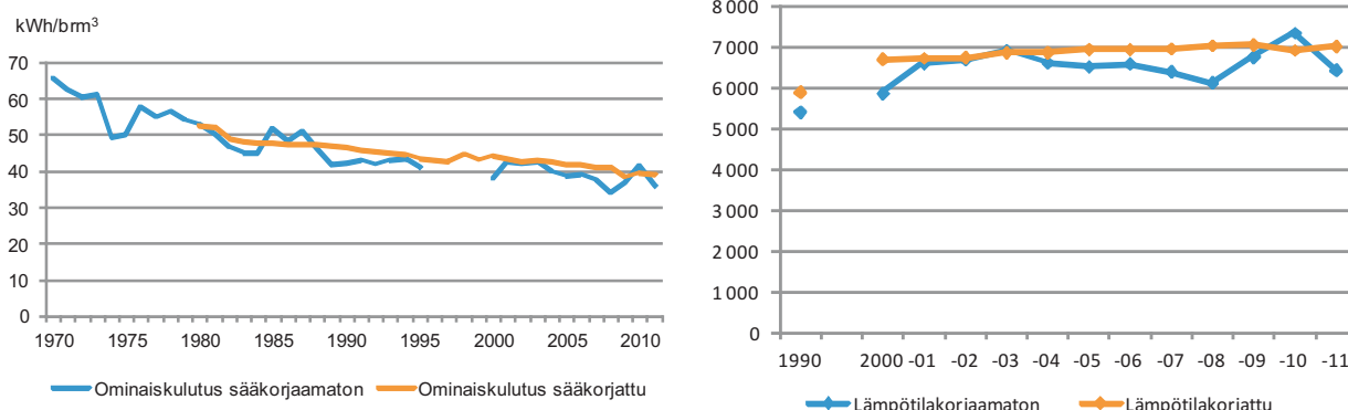
Kuviot 6.7.2–3. Helsingin kaukolämmitteisen rakennuskannan ominaislämmönkulutus 1970–2011 sekä kokonaiskulutus 1990–2011
