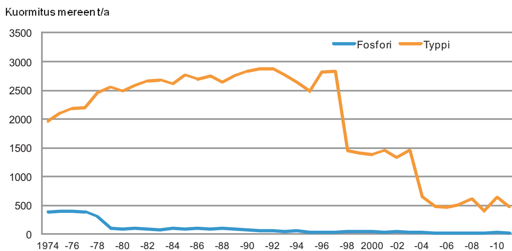
Kuvio 6.8.5. Viikinmäen puhdistamolta mereen johdettu typpi- ja fosforikuormitus 1974-2011
