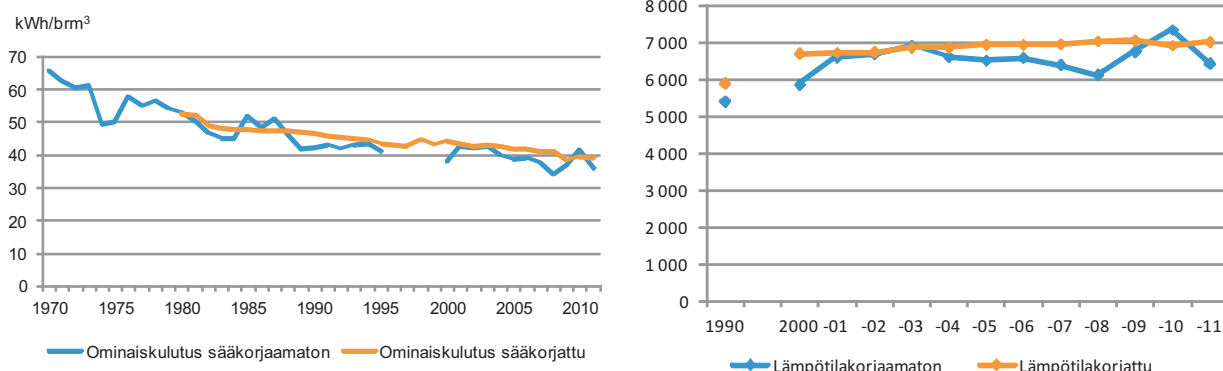
Kuviot 6.8.2–3. Helsingin kaukolämmitteisen rakennuskannan ominaislämmönkulutus 1970–2011 sekä kokonaiskulutus 1990–2011
