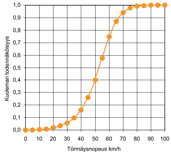
Kuva 10.1.6 Jalankulkijan kuoleman todennäköisyyden riippuvuus henkilöauton törmäysnopeudesta
