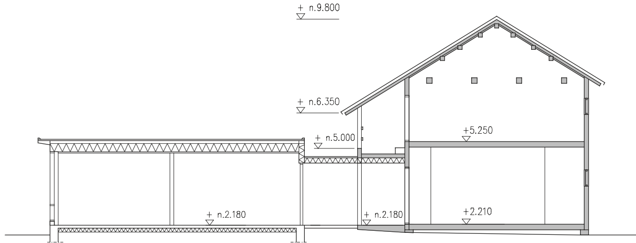
LEIKKAUS A-A
