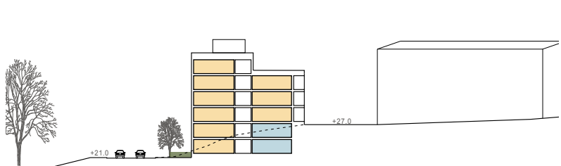
C-C Leikkaus 1:1000
