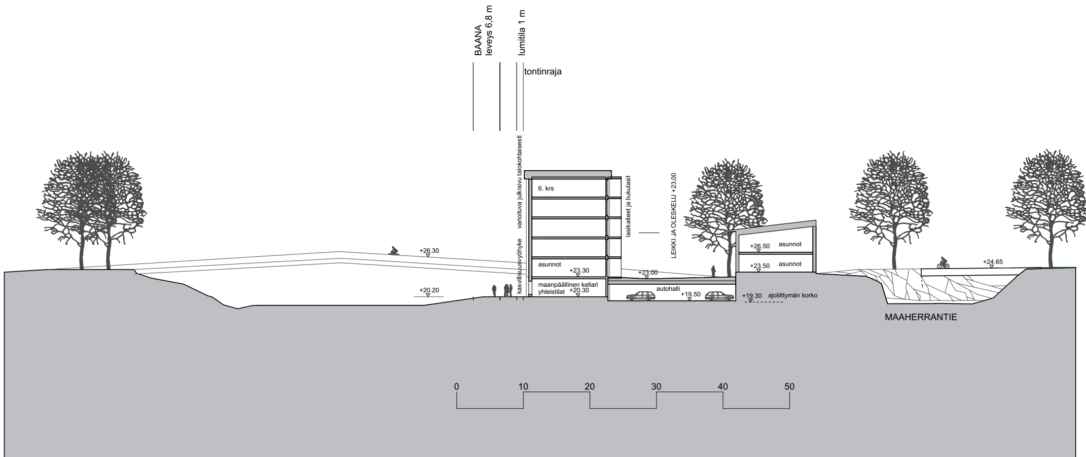
POIKKILEIKKAUS 15.11. 2016
