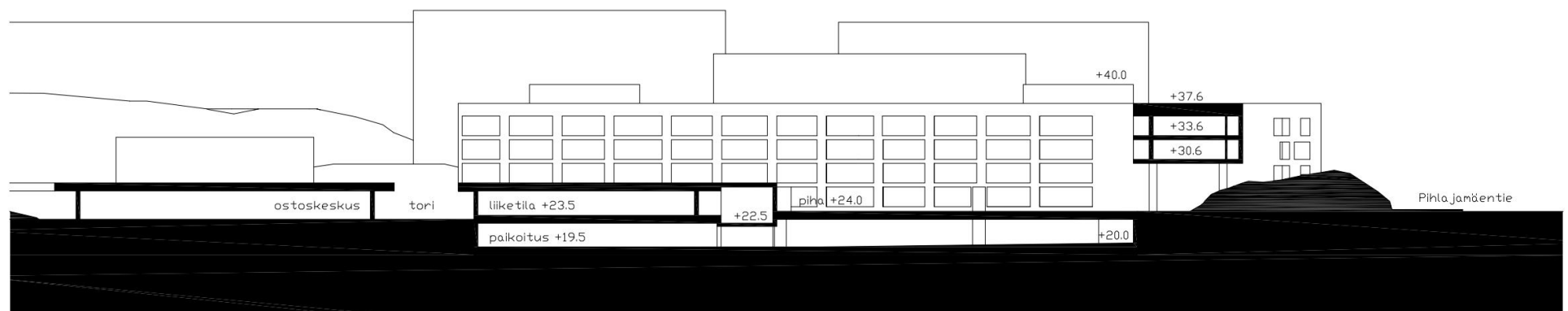
Leikkaus B
