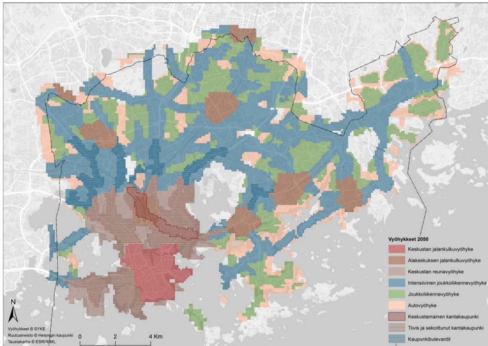
2 Liikkumisvyöhykkeet 2050 tilanteessa. Lähde: SYKE, Keko-hanke
