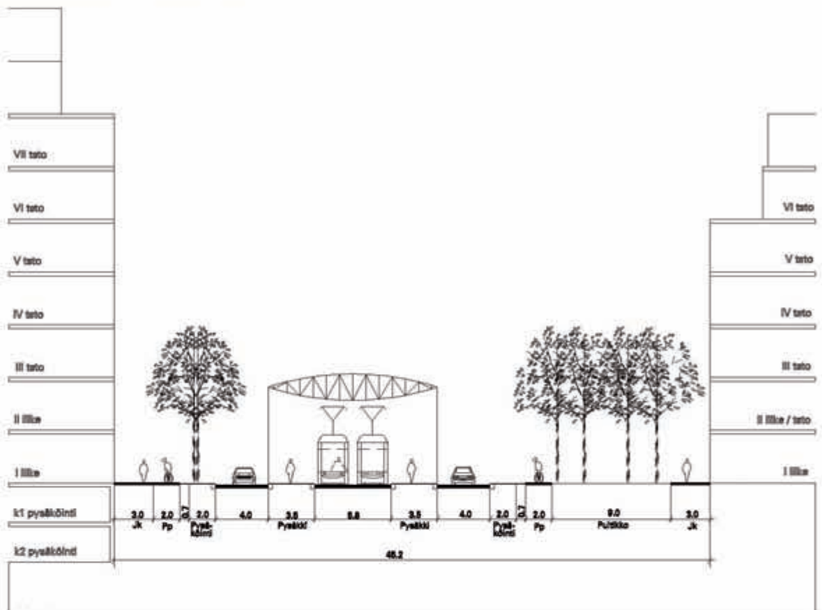
Katupoikkileikkaus 5 - Atlantinkatu, keskus pysäkki
