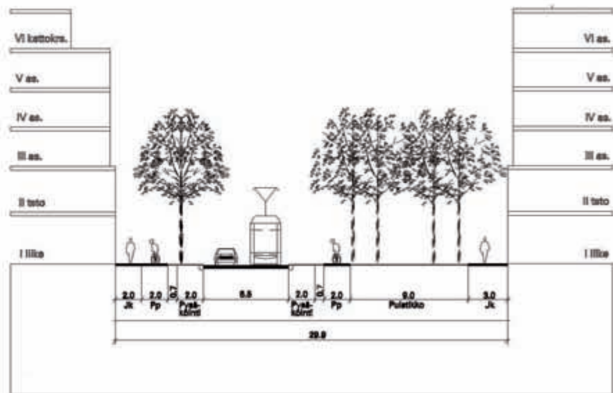
Katupoikkileikkaus 4 - Atlantinkatu
