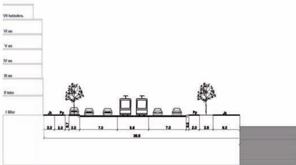
Katupoikkileikkaus 1 - Jätkäsaarenlaituri
