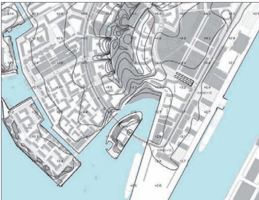
ylh. Jätkäsaaren nykyisiä korkeusasemia alh. Jätkäsaaren tulevia korkeusasemia
