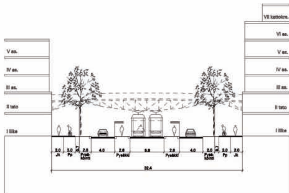
Katupoikkileikkaus 3 - Välimerenkatu, pysäkki
