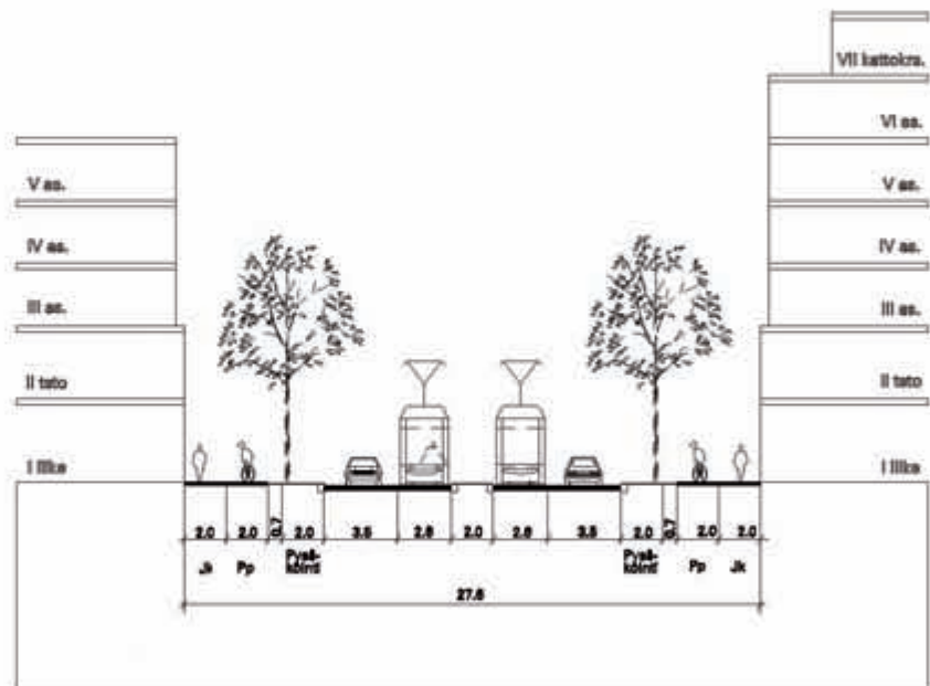
Katupoikkileikkaus 2 - Välimerenkatu
