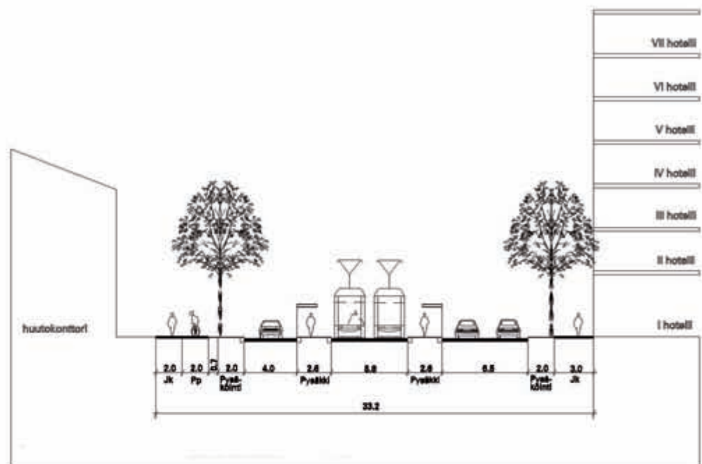
Katupoikkileikkaus 9 - Valtamerenkatu, pysäkki Välimerenkadun liittymässä
