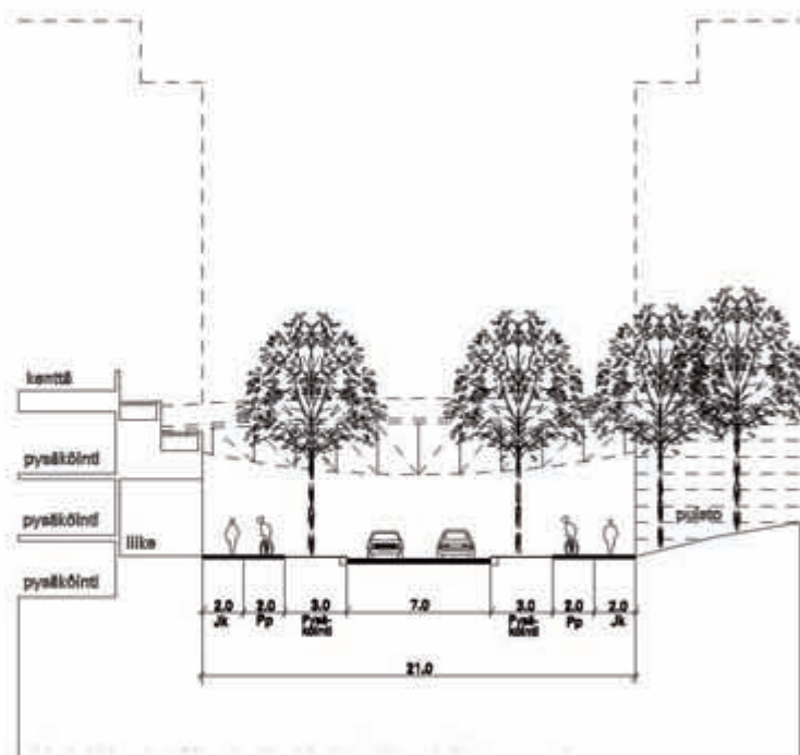
Katupoikkileikkaus 7 - Länsisatamankatu välillä Atlantinkatu - Valtamerenkatu
