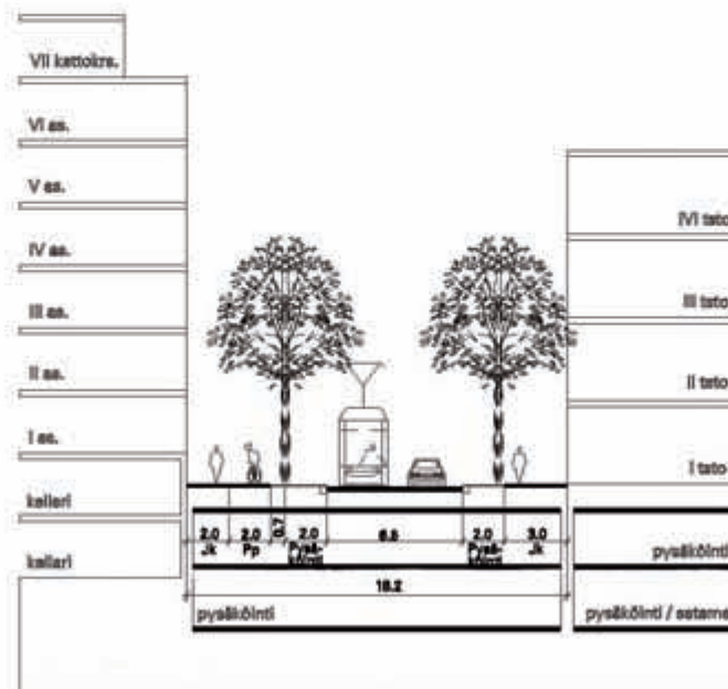
Katupoikkileikkaus 10 - Valtamerenkatu, sataman liittymän jälkeen
