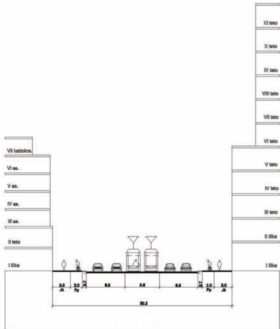
Katupoikkileikkaus 6- Länsisatamankatu välillä Välimerenkatu - Atlantinkatu
