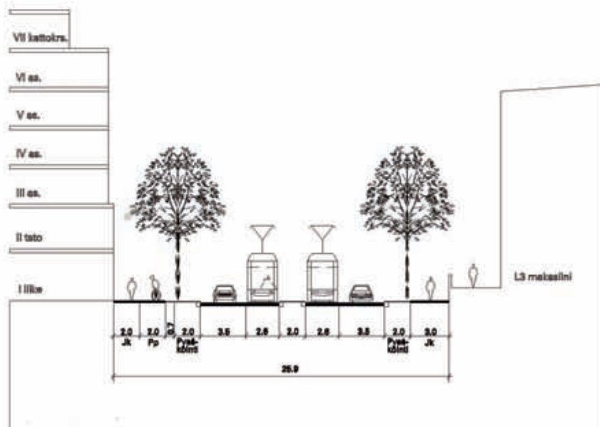
Katupoikkileikkaus 8 - Valtamerenkatu
