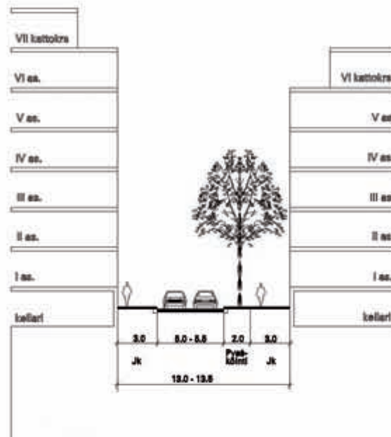
Katupoikkileikkaus 11 - tonttikadut
