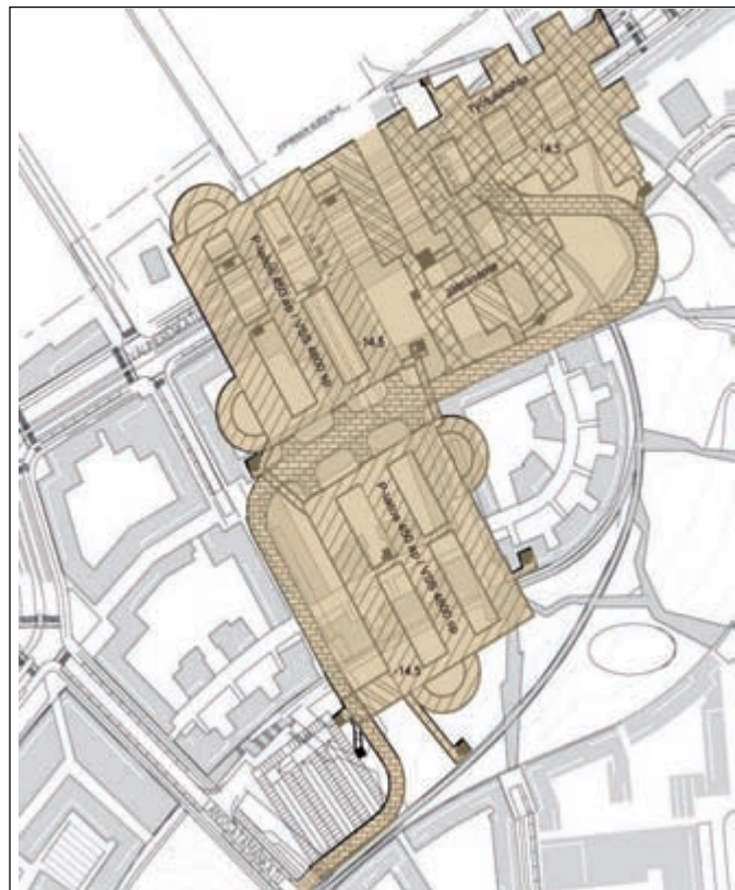
ylh. Jätkäsaaren kalliitilojen alustava suunnitelma alh. Alueelliseen pysäköintilaitosjärjestelmään kuuluvat autopaikat. Saukonrannassa ja -nokassa paikoitus järjestetään tontti- tai korttelikohtaisesti.
