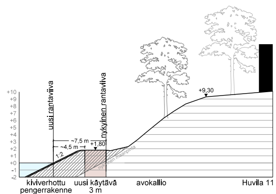
Tutkielma Töölönlahden 3 m leveän rantaraitin tilavaatimuksista Linnunlaulun huvilan 11 kohdalla. Maisema-arkkitehtitoimisto Näkymä Oy
