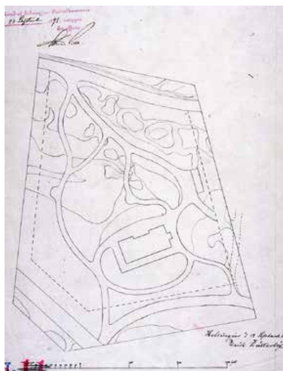
Sokeainkodin puutarhasuunnitelman laatija oli Erik Zätterlöf. Förslag till planering vid Blindhemmet i Djurgården No 7, Helsingfors 12 September 1893. HKA
