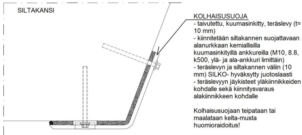
Kuva 3. Esimerkki jälkiasennettavasta kolhaisusuojusta
