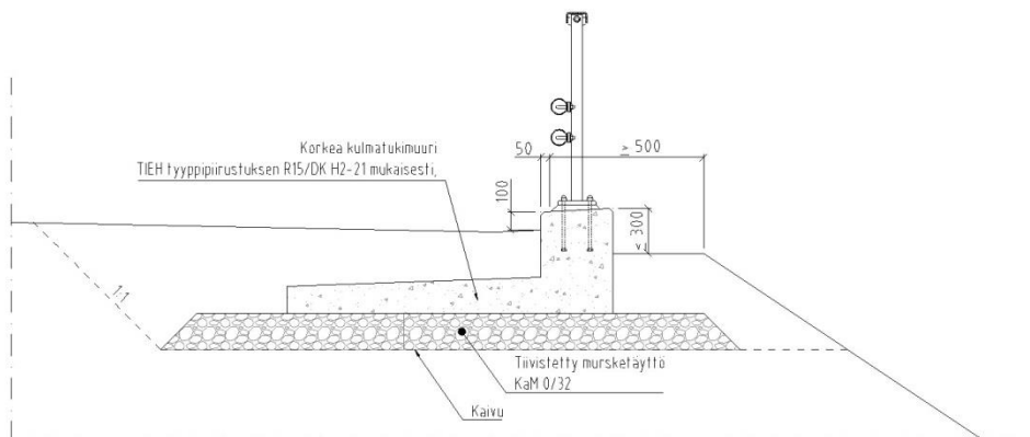
Kuva 6. Kulmatukimuuirelementti sillan taustalla ja 2-putkikaide. Kaidetyyppi suunnitellaan kohdekohtaisesti.
