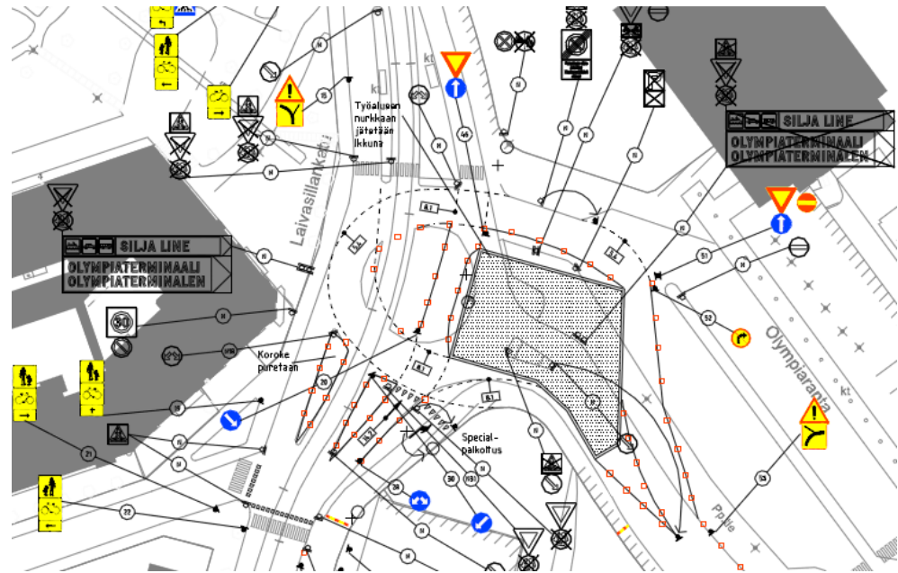
Kuva 9. Ote liikenteenohjaussuunnitelmasta
